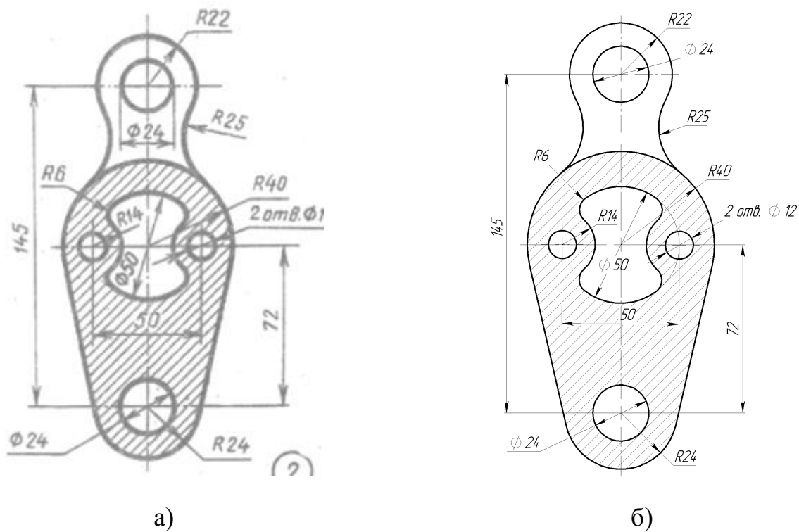
Рисунок 2. Подвеска: а – задание; б – готовый эскиз детали
