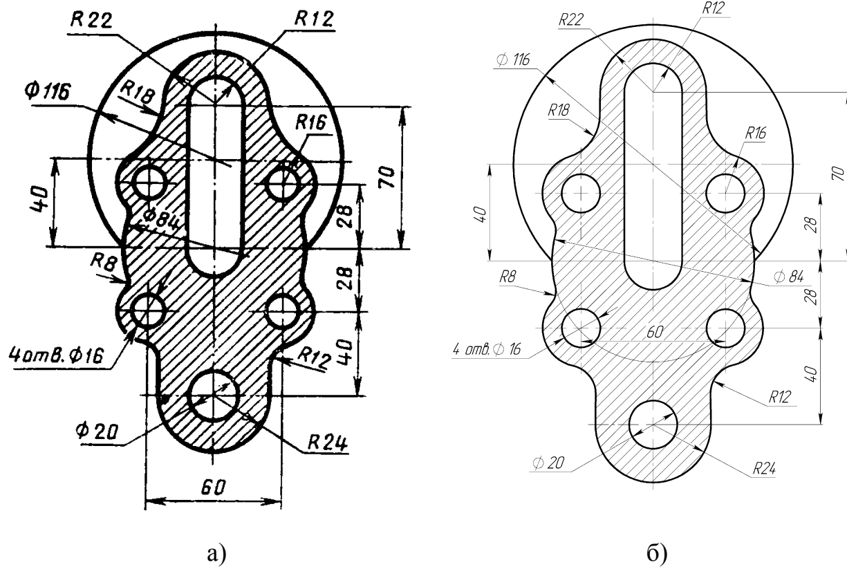
Рисунок 2. Крышка: а – задание; б – готовый эскиз детали
