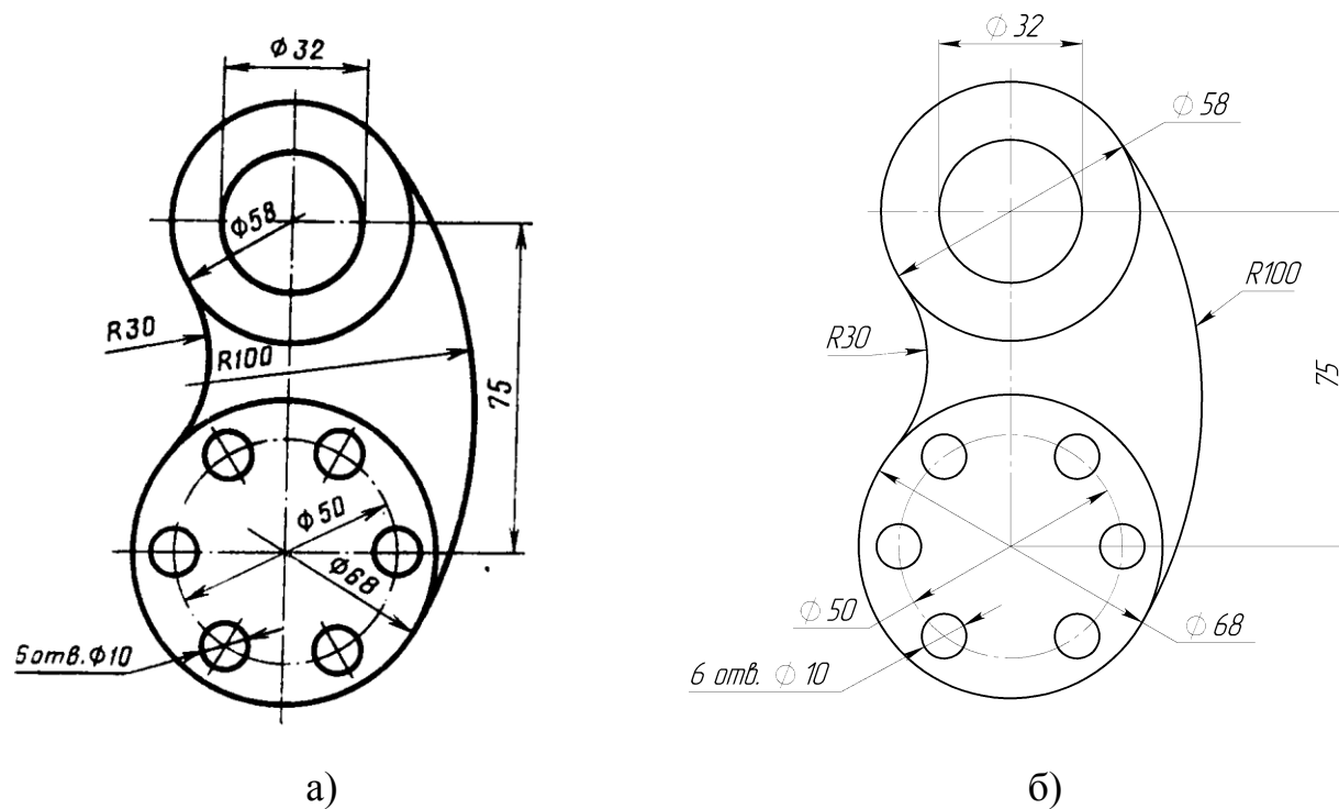
Рисунок 1. Кронштейн: а – задание; б – готовый эскиз детали
