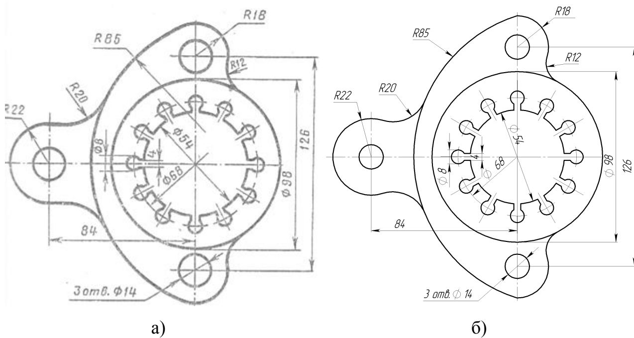
Рисунок 1. Проушина: а – задание; б – готовый эскиз детали
