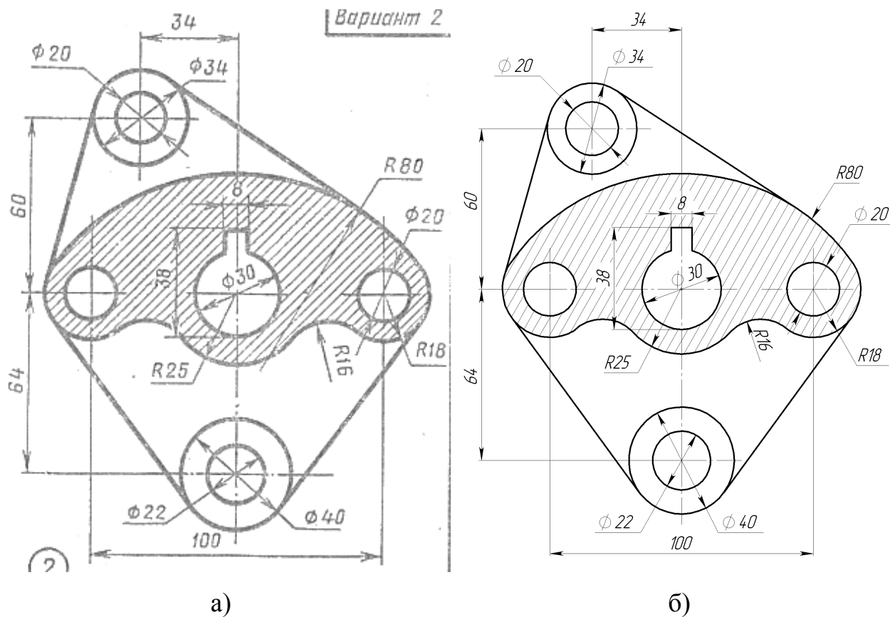
Рисунок 2. Рычаг: а – задание; б – готовый эскиз детали
