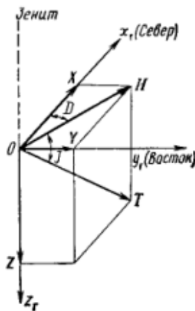
Рис.1. Элементы МПЗ
