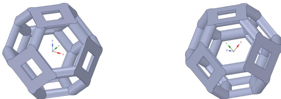
Рис.1.5.5.6. Внешний вид ячейки типа 6 до и после поворота локальных осей
