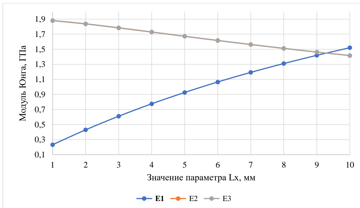
Рис.1.5.3.8. Зависимость значений модулей Юнга от параметра L_x для ячейки типа 1
