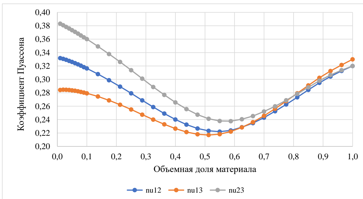
Рис.1.5.2.15. Зависимость значений коэффициента Пуассона от объемной доли материала для ячейки типа 4
