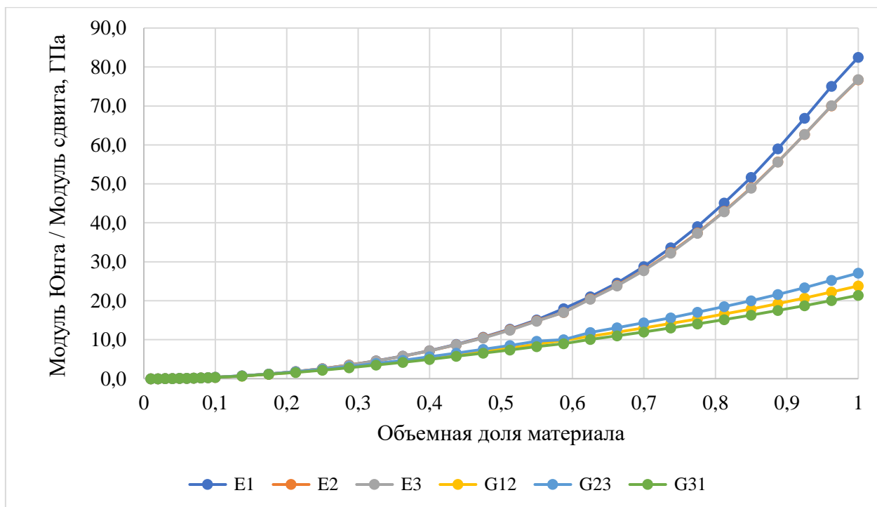
Рис.1.5.2.12. Зависимость значений модулей Юнга и модулей сдвига от объемной доли материала для ячейки типа 3
