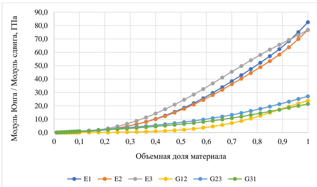
Рис.1.5.2.18. Зависимость значений модулей Юнга и модулей сдвига от объемной доли материала для ячейки типа б
