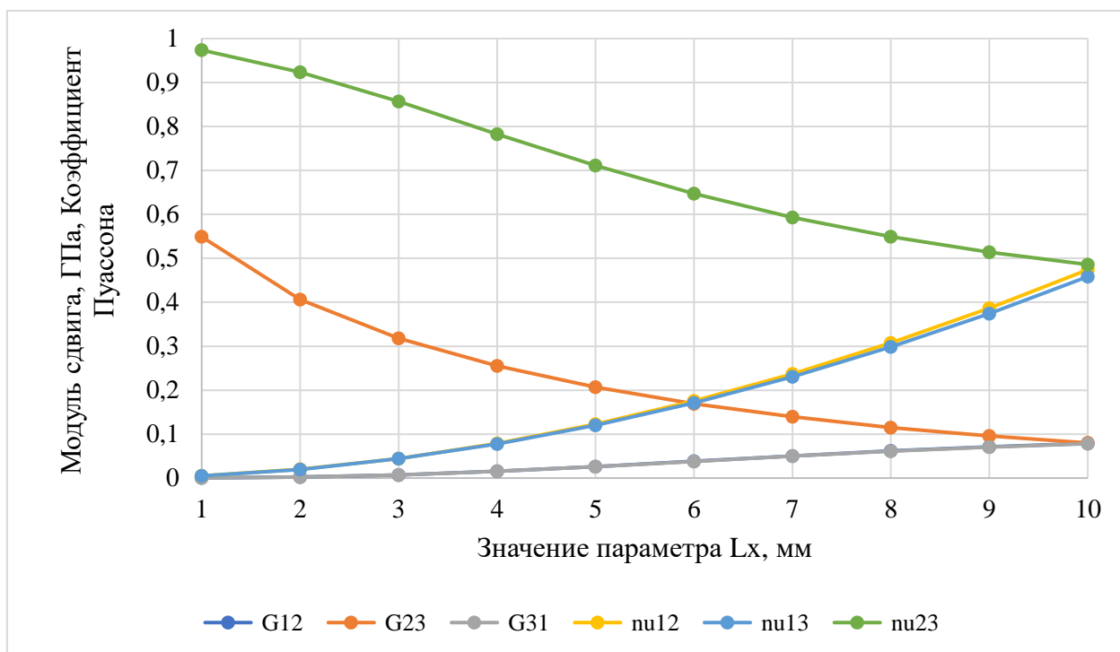
Рис.1.5.3.13. Зависимость значений модулей сдвига и коэффициентов Пуассона от параметра L_x для ячейки типа 3
