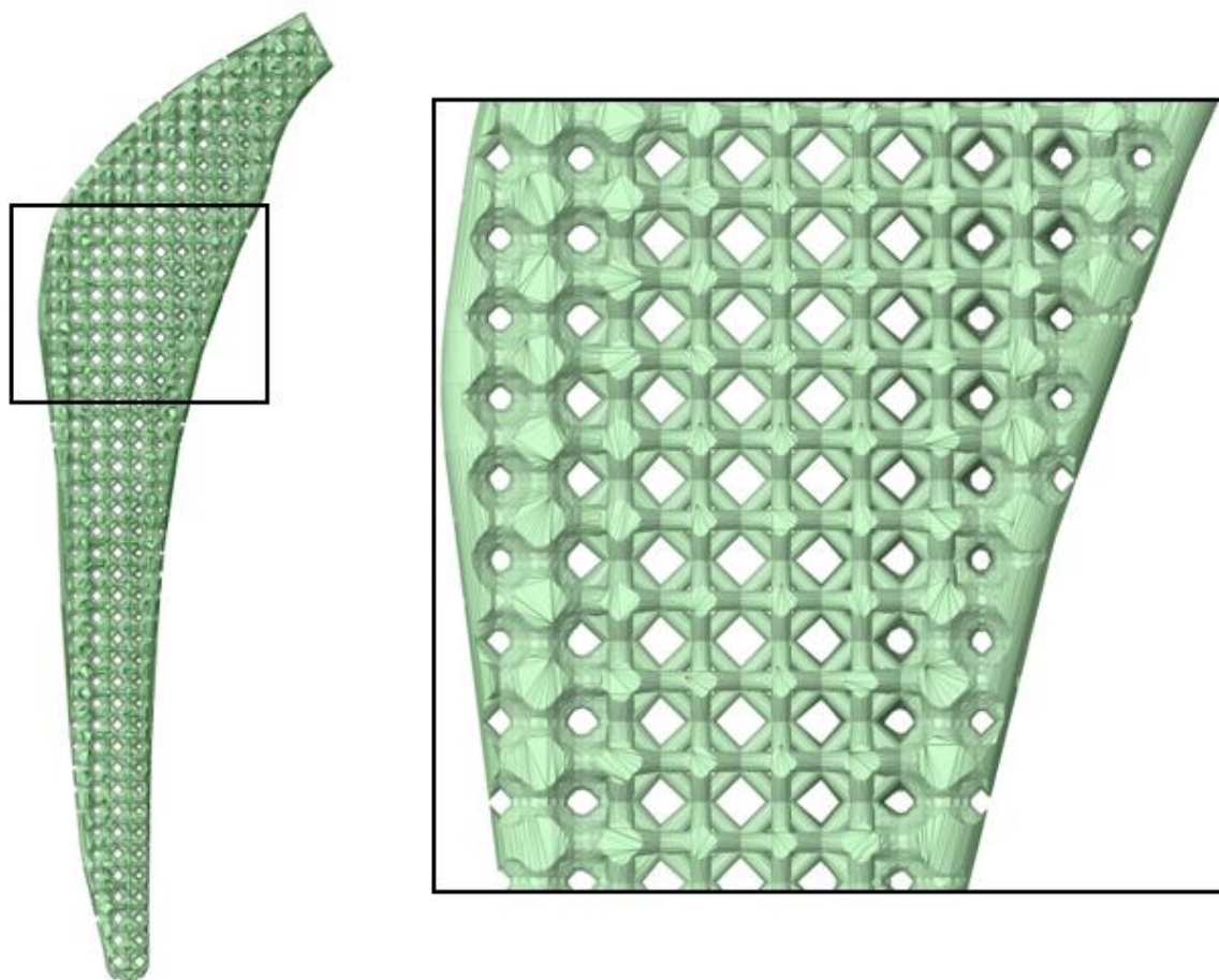
Рис.2.3.2. Внешний вид геометрии компонента эндопротеза, включающей в себя решетчатые структуры
