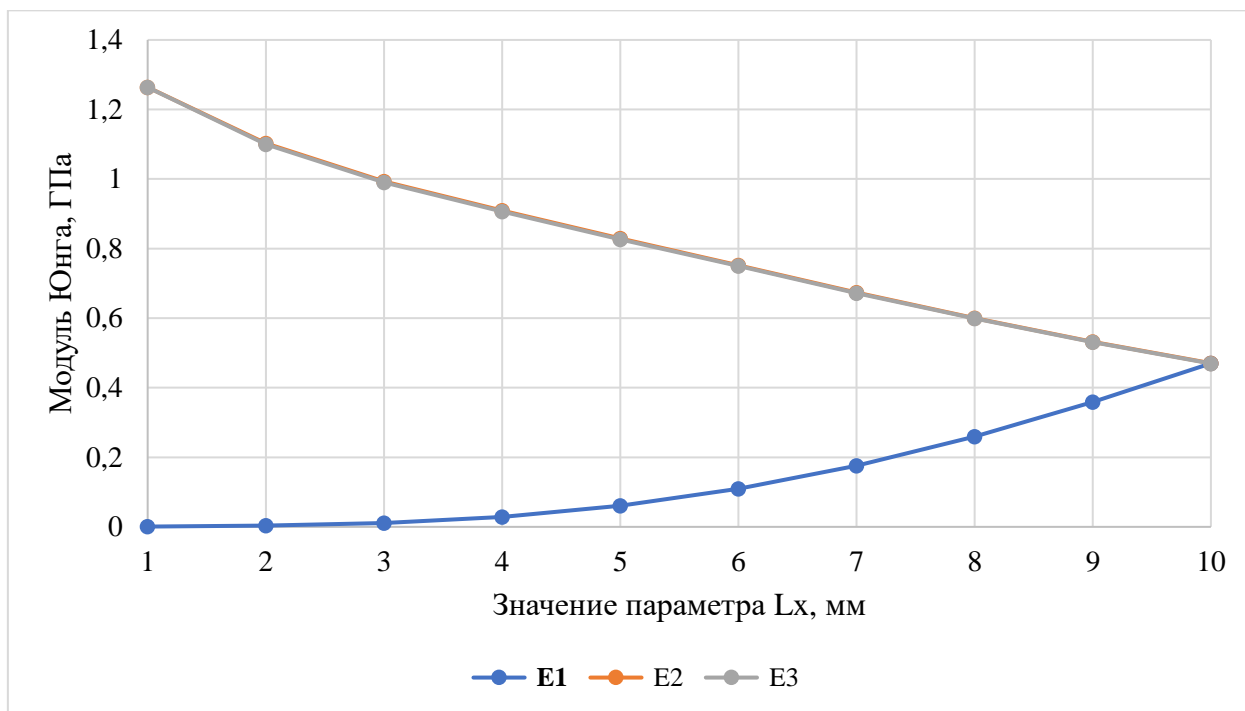
Рис.1.5.3.14. Зависимость значений модулей Юнга от параметра L_x для ячейки типа 4
