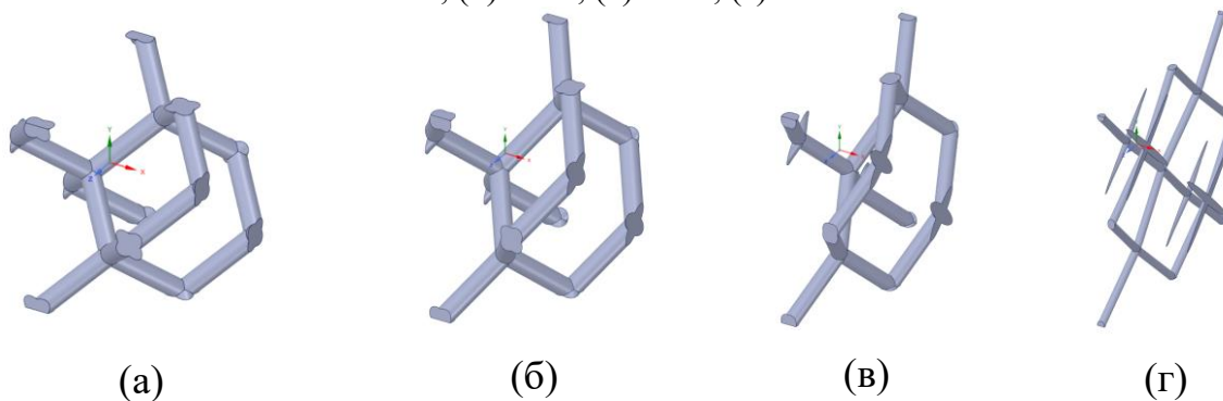
Рис.1.5.3.3. Внешний вид ячейки типа 3 при изменении геометрического размера L_x : (а) 10 мм, (б) 7 мм, (в) 4 мм, (г) 1 мм
