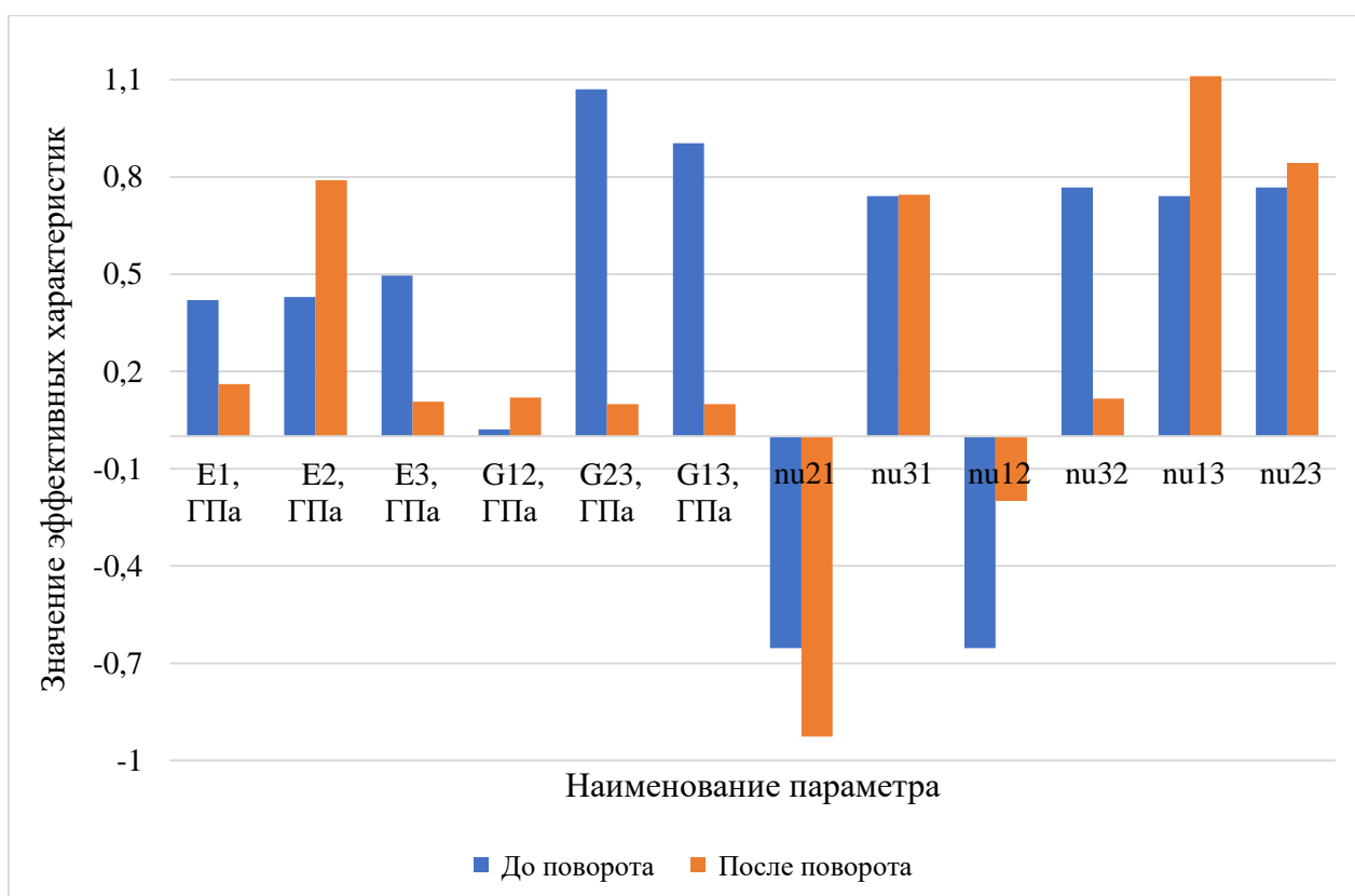
Рис.1.5.5.12. Значения эффективных характеристик до и после поворота локальных осей для элементарной ячейки типа 5
