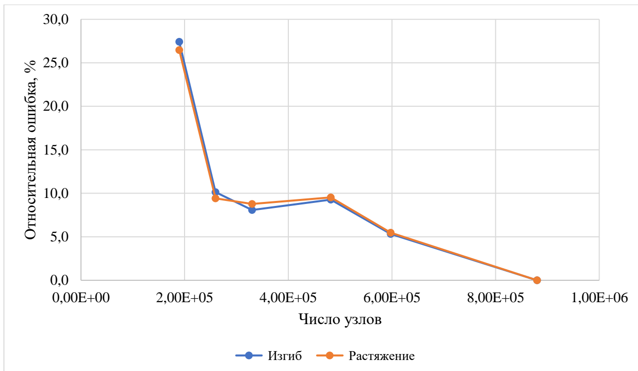
Рис.2.4.2. Графическое представление сеточной сходимости
