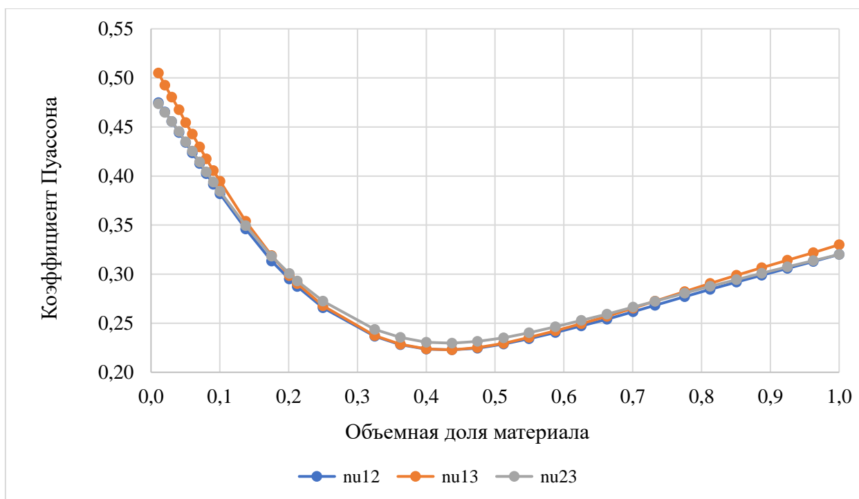
Рис.1.5.2.21. Зависимость значений коэффициента Пуассона от объемной доли материала для ячейки типа 7
