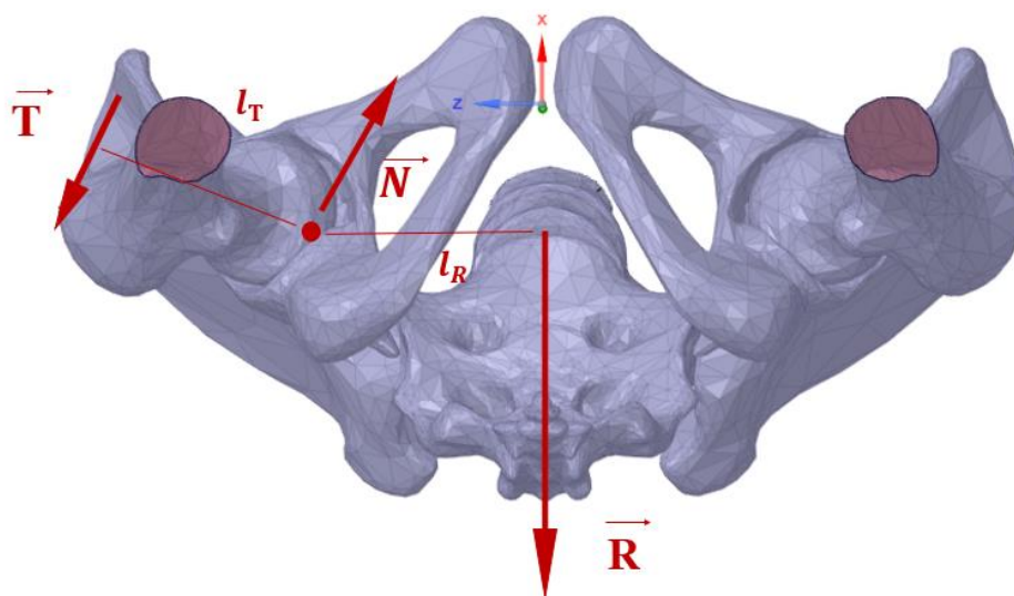
Рис.2.2.2.2. Схема нагружения модели таза. 2 сценарий нагружения
