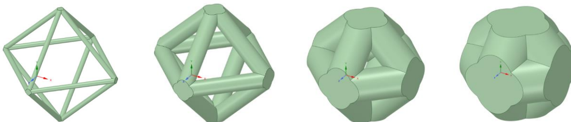
Рис. 1.5.2.3. Внешний вид ячейки типа 3 при различных значениях объемной доли материала: (а) 0,01; (б) 0,1; (в) 0,4; (г) 0,7
