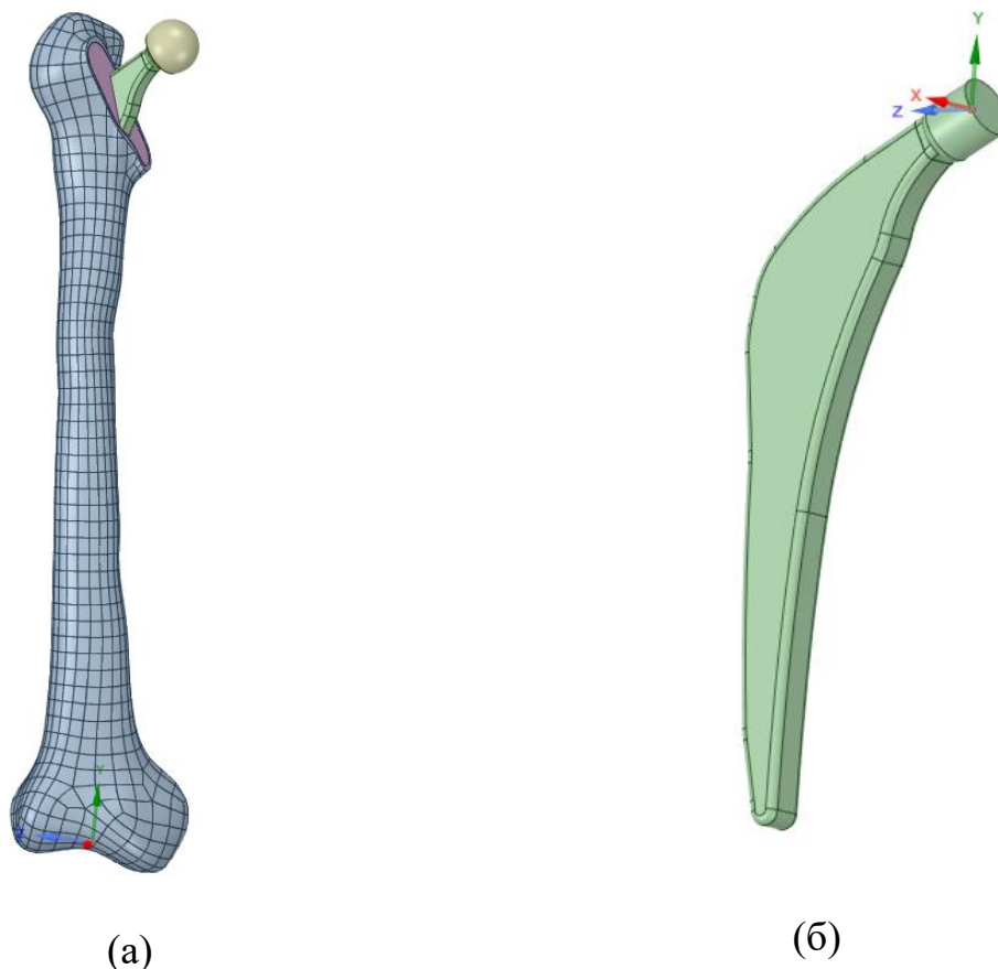
Рис.2.1.1. Внешний вид геометрии эндопротеза тазобедренного сустава, (а) общий вид, (б) крупное представление элемента эндопротеза
