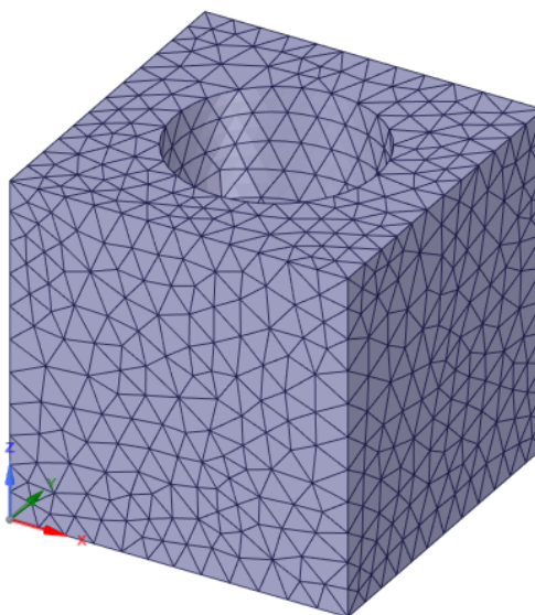
Рис.1.3.2. Вид конечно-элементной модели элементарной ячейки простейшего вида
