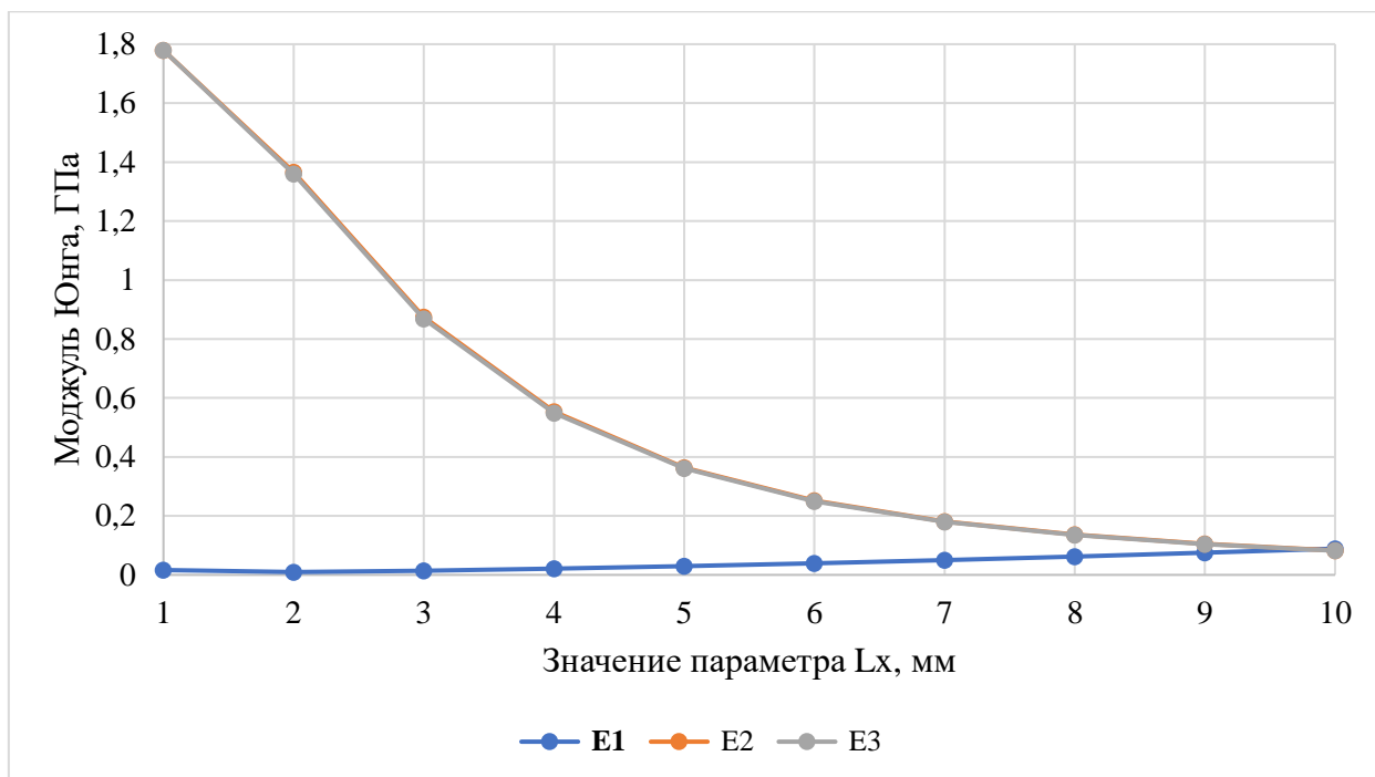
Рис.1.5.3.18. Зависимость значений модулей Юнга от параметра L_x для ячейки типа 6
