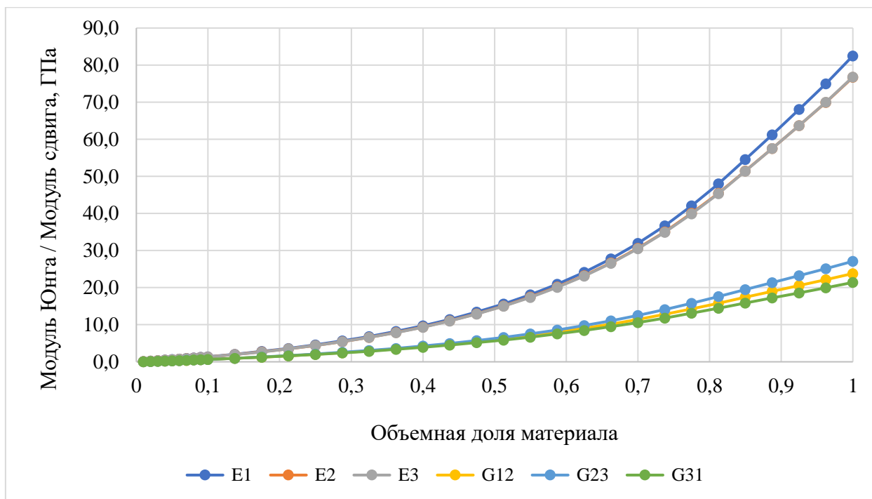
Рис.1.5.2.10. Зависимость значений модулей Юнга и модулей сдвига от объемной доли материала для ячейки типа 2
