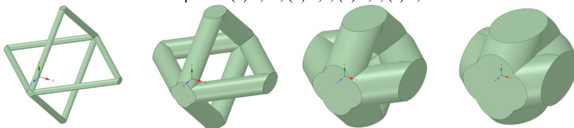
Рис. 1.5.2.5. Внешний вид ячейки типа 5 при различных значениях объемной доли материала: (а) 0,01; (б) 0,1; (в) 0,4; (г) 0,7
