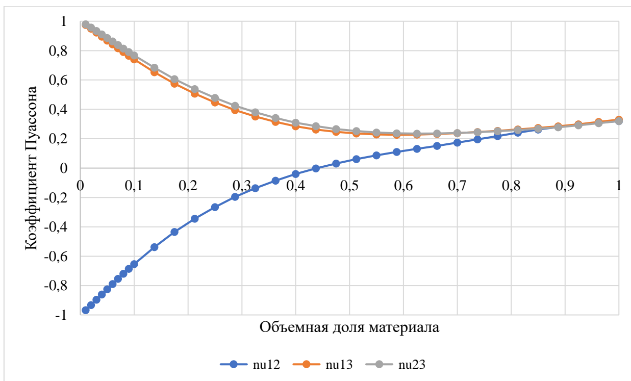
Рис.1.5.2.19. Зависимость значений коэффициента Пуассона от объемной доли материала для ячейки типа б
