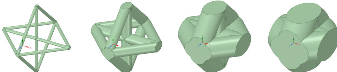
Рис. 1.5.2.4. Внешний вид ячейки типа 4 при различных значениях объемной доли материала: (а) 0,01; (б) 0,1; (в) 0,4; (г) 0,7
