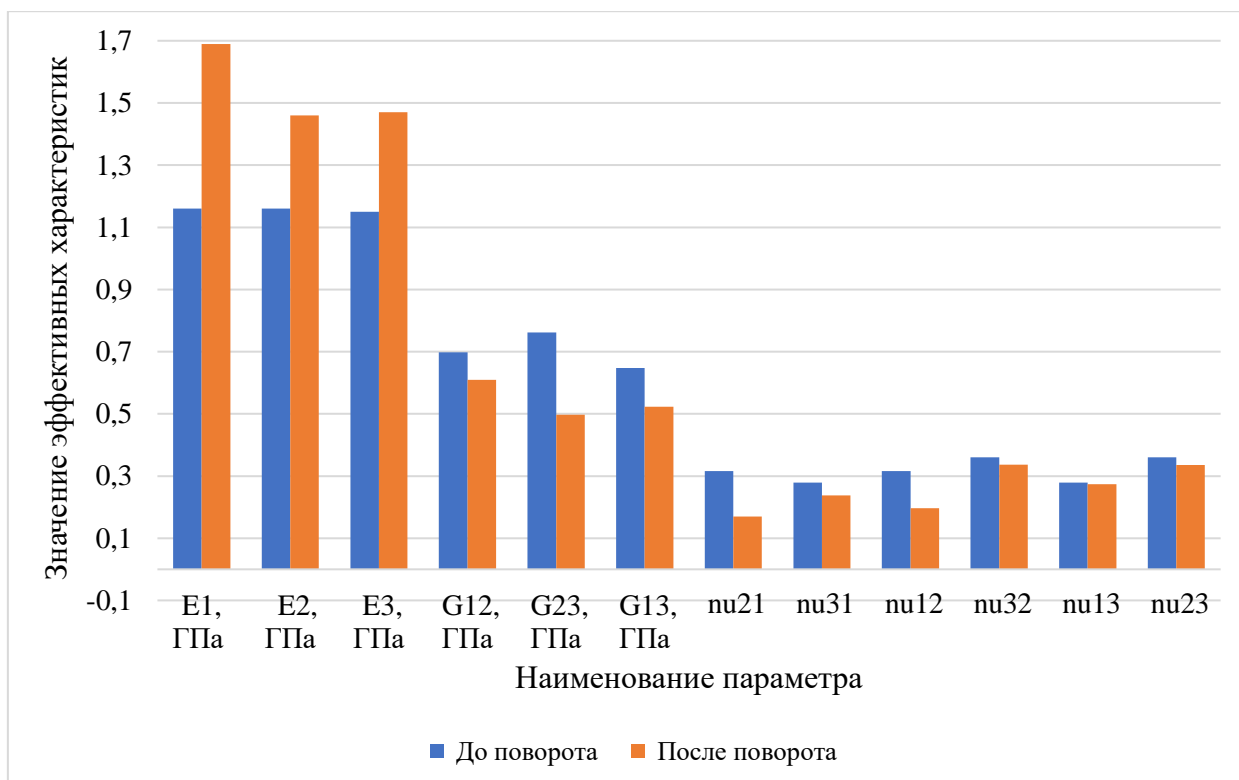
Рис.1.5.5.10. Значения эффективных характеристик до и после поворота локальных осей для элементарной ячейки типа 3
