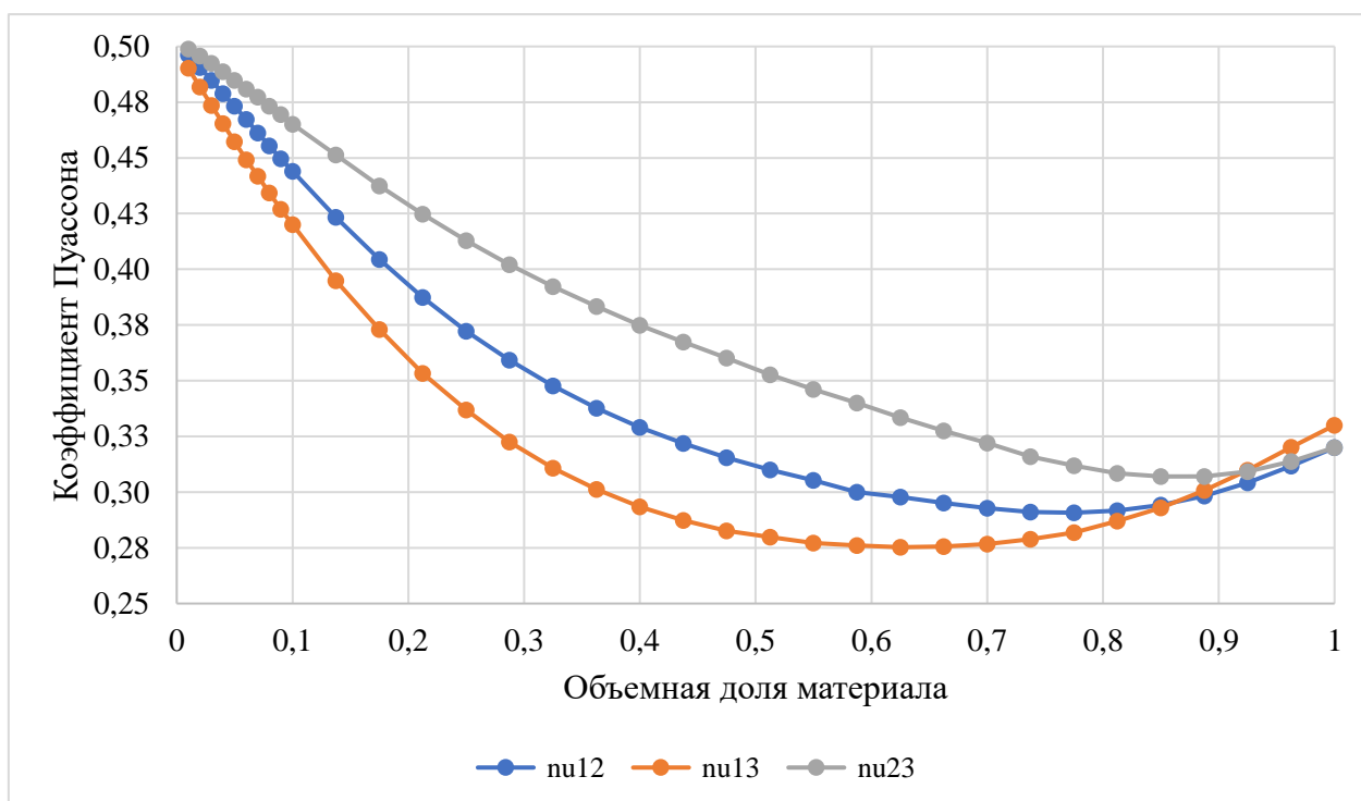
Рис.1.5.2.13. Зависимость значений коэффициента Пуассона от объемной доли материала для ячейки типа 3
