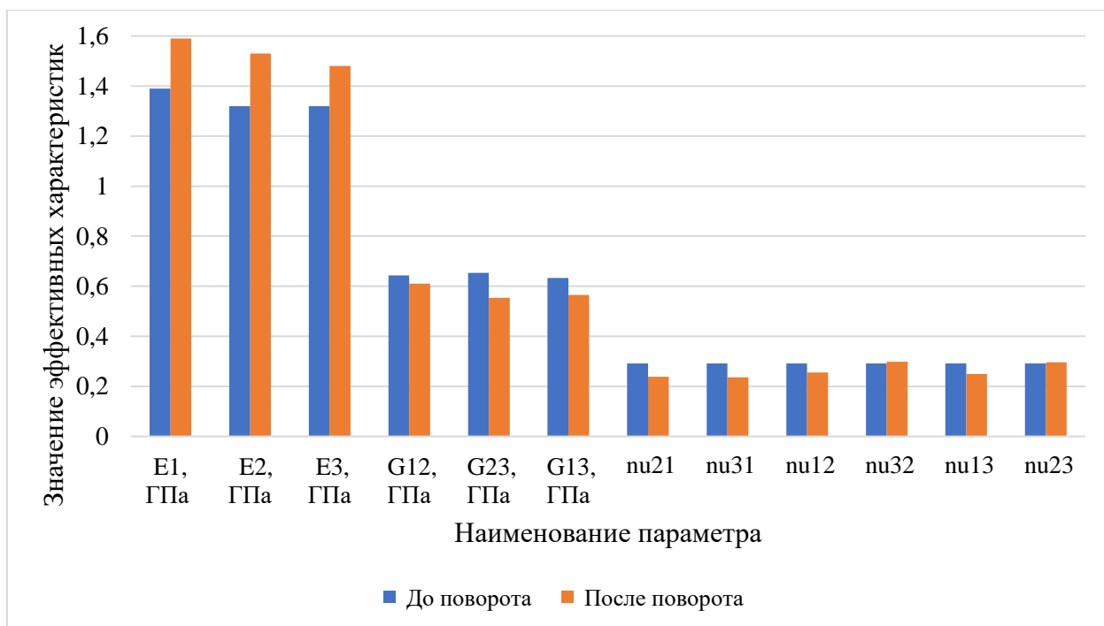
Рис.1.5.5.9. Значения эффективных характеристик до и после поворота локальных осей для элементарной ячейки типа 2
