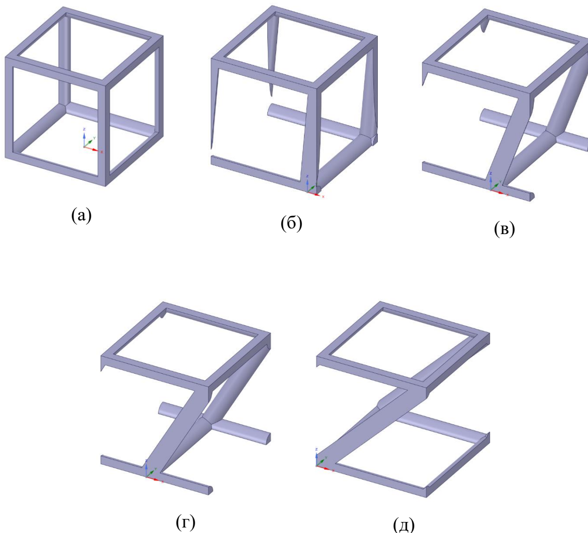
Рис.1.5.4.1. Внешний вид элементарной ячейки типа 1 при изменении угла между стержнями: (а) 90 градусов; (б) 85 градусов; (в) 70 градусов; (г) 60 градусов; (д) 45 градусов
