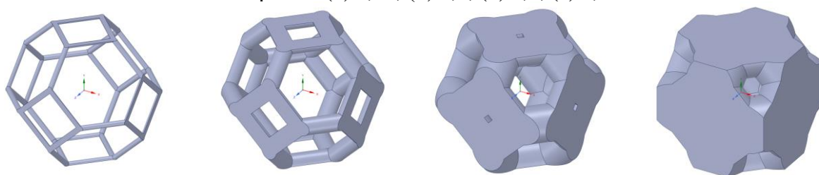
Рис. 1.5.2.6. Внешний вид ячейки типа 6 при различных значениях объемной доли материала: (а) 0,01; (б) 0,1; (в) 0,4; (г) 0,7
