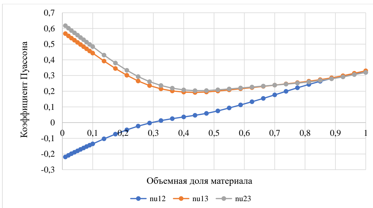
Рис.1.5.2.17. Зависимость значений коэффициента Пуассона от объемной доли материала для ячейки типа 5
