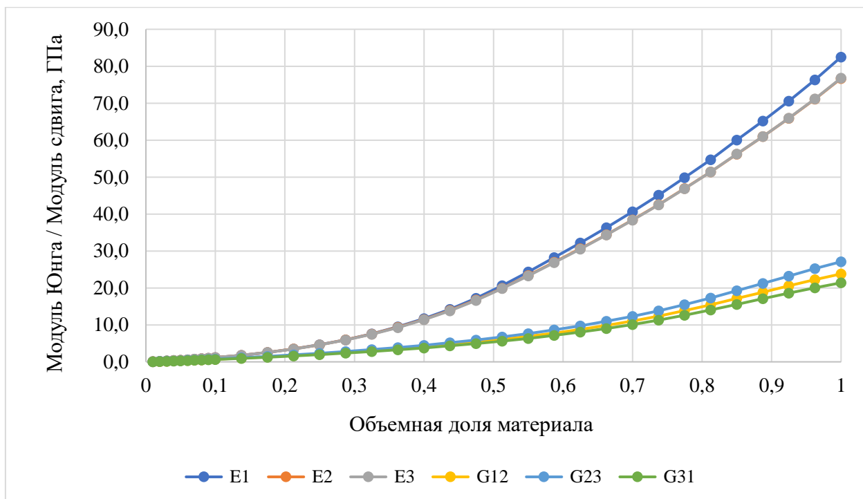
Рис.1.5.2.14. Зависимость значений модулей Юнга и модулей сдвига от объемной доли материала для ячейки типа 4
