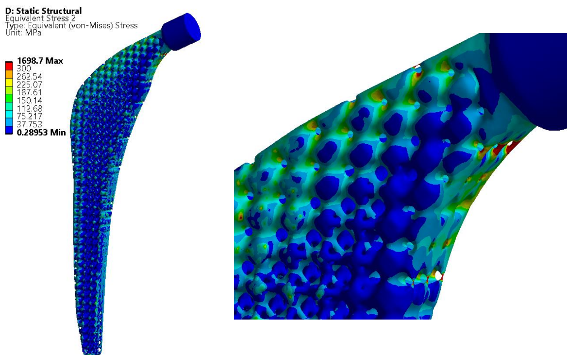
Рис.2.4.5. Эквивалентные напряжения (по Мизесу) компонента эндопротеза. 2 сценарий нагружения
