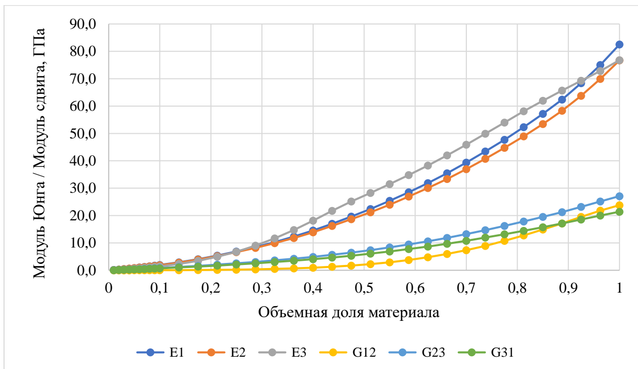
Рис.1.5.2.16. Зависимость значений модулей Юнга и модулей сдвига от объемной доли материала для ячейки типа 5
