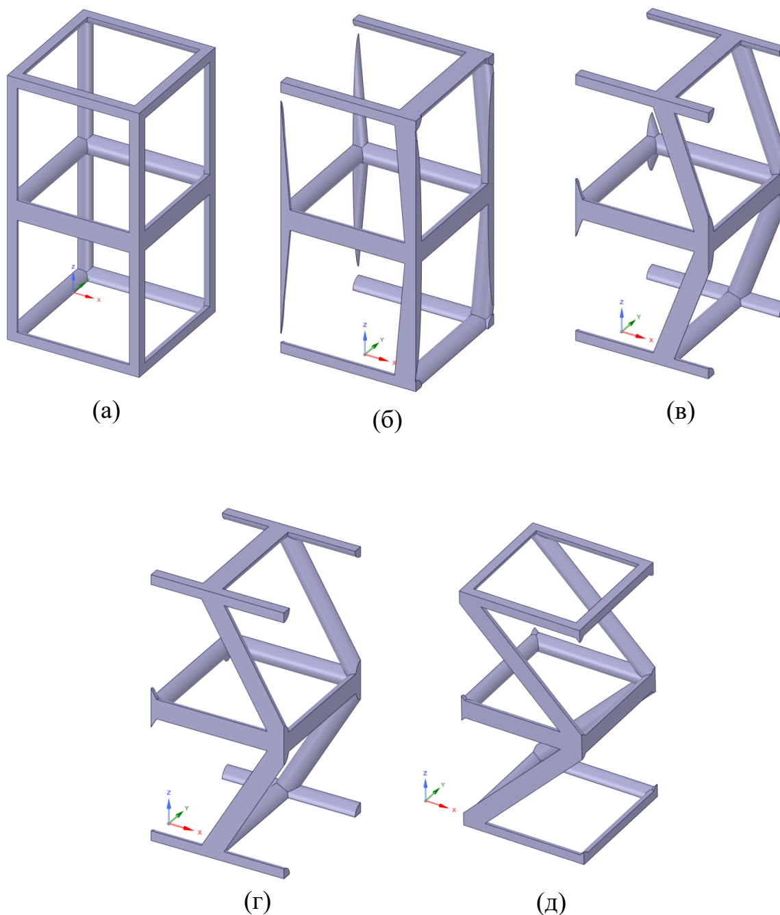
Рис.1.5.4.2. Внешний вид элементарной ячейки типа 1 при изменении угла между стержнями после симметричного отражения: (а) 90 градусов; (б) 85 градусов; (в) 70 градусов; (г) 60 градусов; (д) 45 градусов
