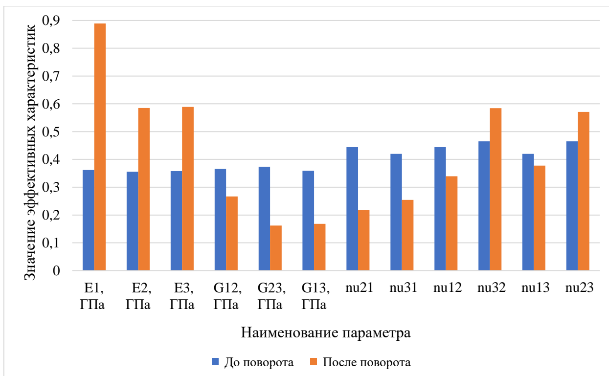
Рис.1.5.5.10. Значения эффективных характеристик до и после поворота локальных осей для элементарной ячейки типа 3
