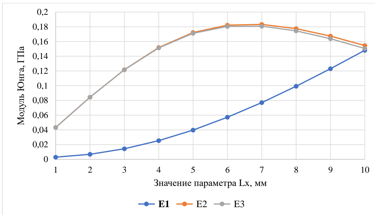
Рис.1.5.3.20. Зависимость значений модулей Юнга от параметра L_x для ячейки типа 7
