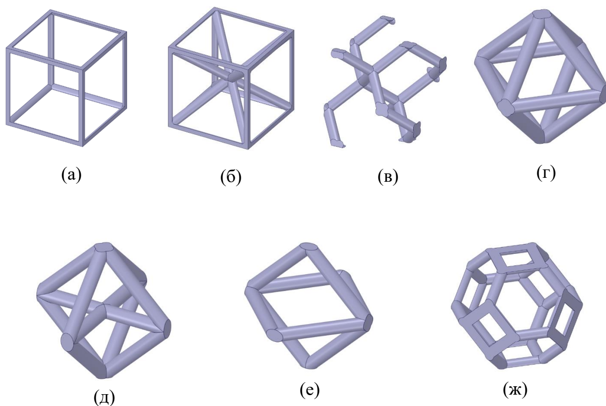
Рис. 1.2.1. Базовые ячейки метаматериалов: (а) ячейка типа 1, (б) ячейка типа 2, (в) ячейка типа 3, (г) ячейка типа 4, (д) ячейка типа 5, (е) ячейка типа 6, (ж) ячейка типа 7
