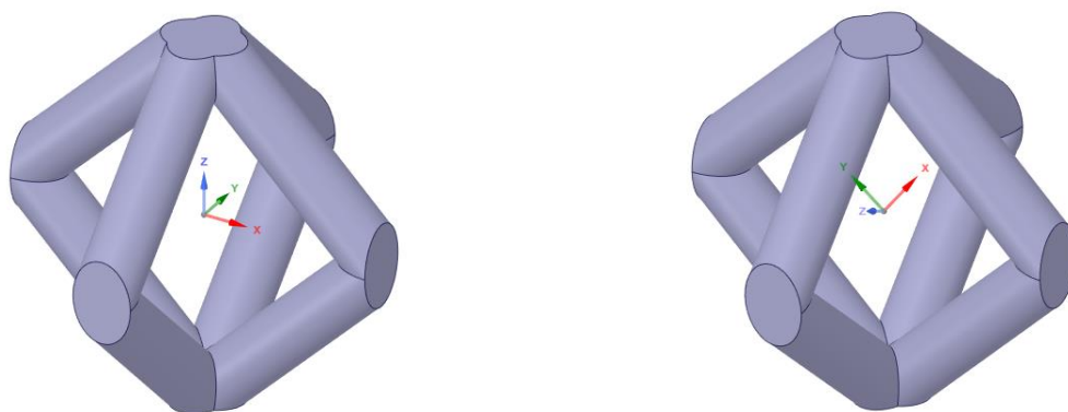
Рис.1.5.5.6. Внешний вид ячейки типа 6 до и после поворота локальных осей
