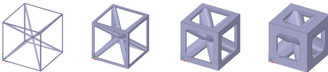
Рис. 1.5.2.1. Внешний вид ячейки типа 1 при различных значениях объемной доли материала: (а) 0,01; (б) 0,1; (в) 0,4; (г) 0,7
