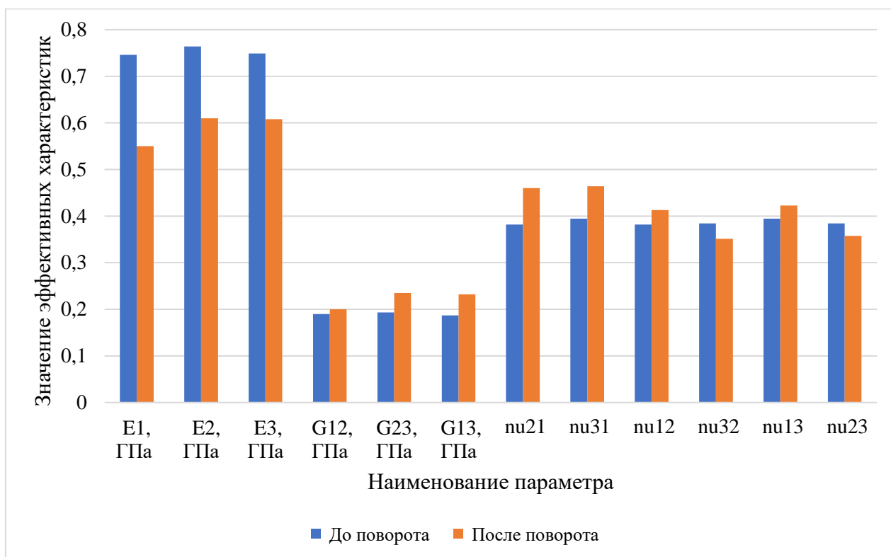
Рис.1.5.5.14. Значения эффективных характеристик до и после поворота локальных осей для элементарной ячейки типа 7
