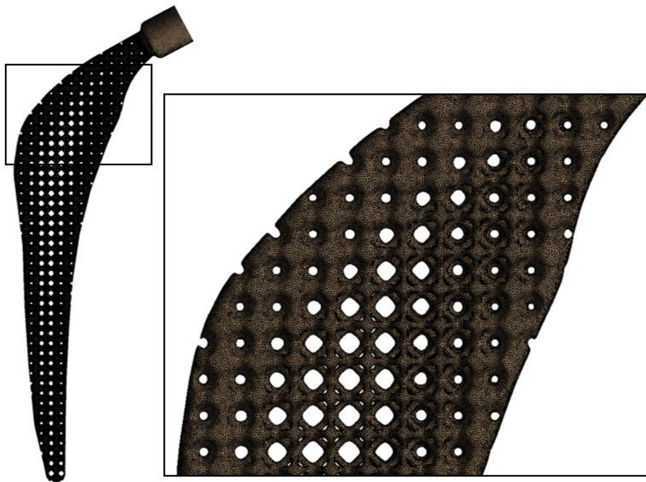
Рис.2.4.3. Конечно-элементная модель компонента эндопротеза
