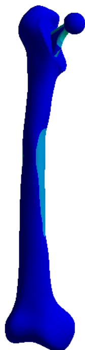
Рис.2.2.1.4. Распределение эквивалентных напряжений (по Мизесу) и модуля вектора перемещений для системы в случае 1 сценария нагружения
