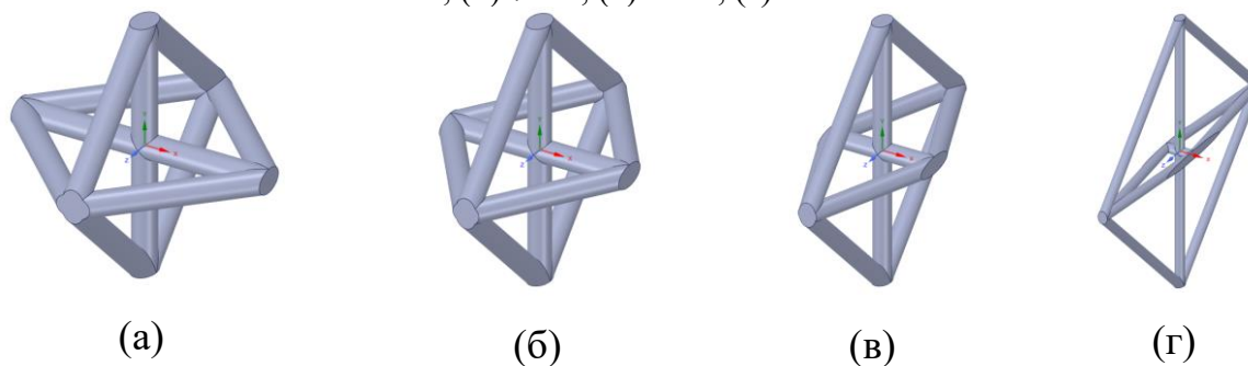
Рис.1.5.3.5. Внешний вид ячейки типа 5 при изменении геометрического размера L_x : (а) 10 мм, (б) 7 мм, (в) 4 мм, (г) 1 мм
