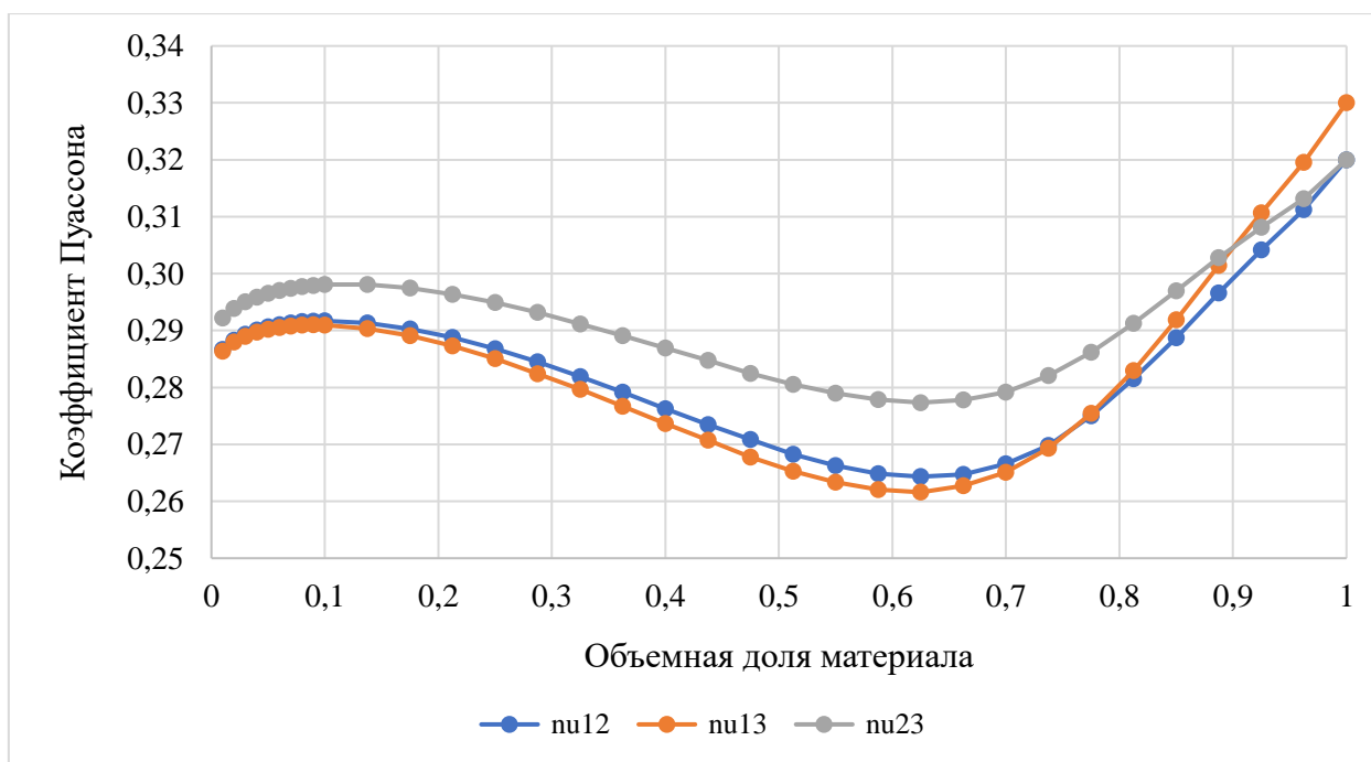
Рис.1.5.2.11. Зависимость значений коэффициента Пуассона от объемной доли материала для ячейки типа 2
