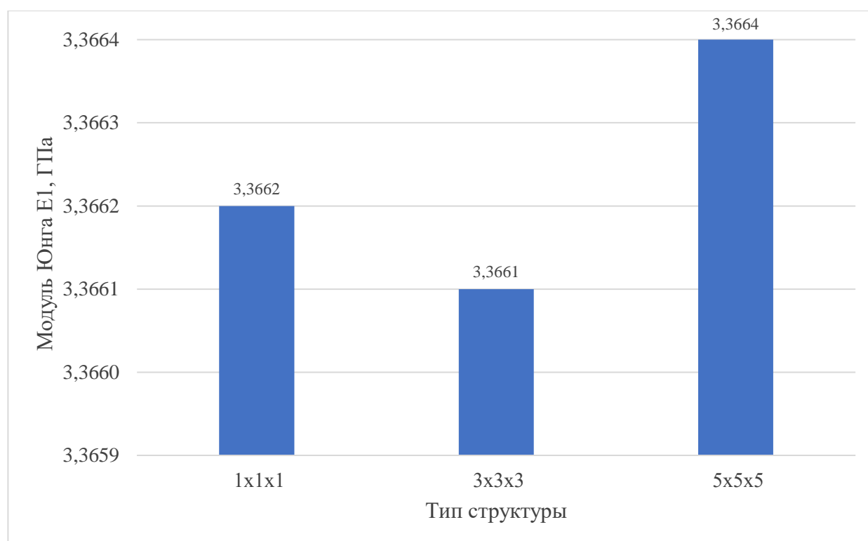
Рис. 1.4.5. Изменение значения модуля Юнга E_1 в зависимости от размера периодической структуры
