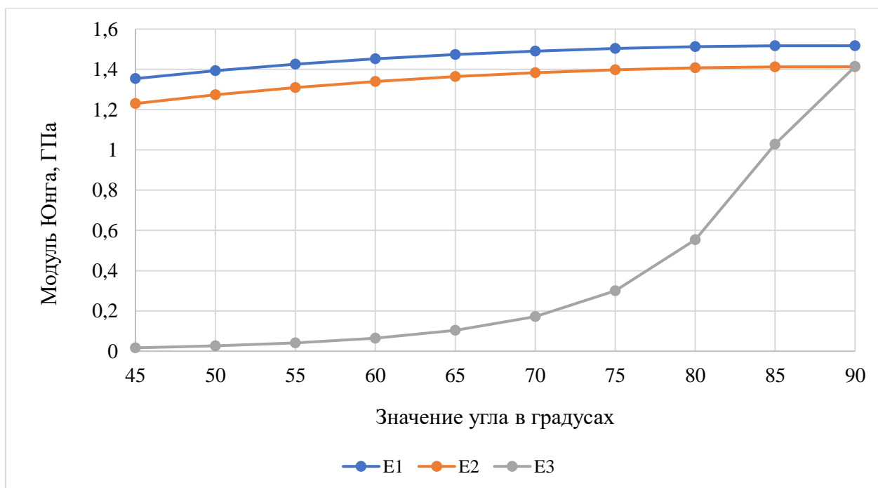
Рис.1.5.4.3. Зависимость модулей Юнга от значения градусной меры угла между стержнями для ячейки типа 1
