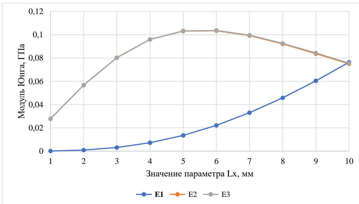
Рис.1.5.3.12. Зависимость значений модулей Юнга от параметра L_x для ячейки типа 3
