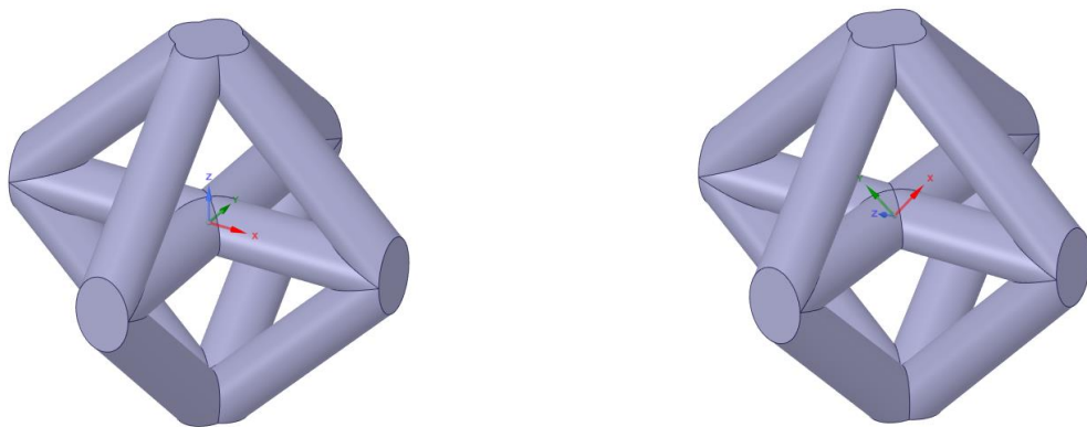
Рис.1.5.5.5. Внешний вид ячейки типа 5 до и после поворота локальных осей
