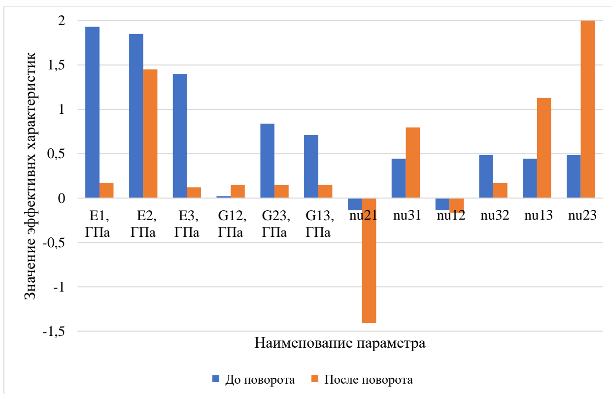
Рис.1.5.5.12. Значения эффективных характеристик до и после поворота локальных осей для элементарной ячейки типа 5
