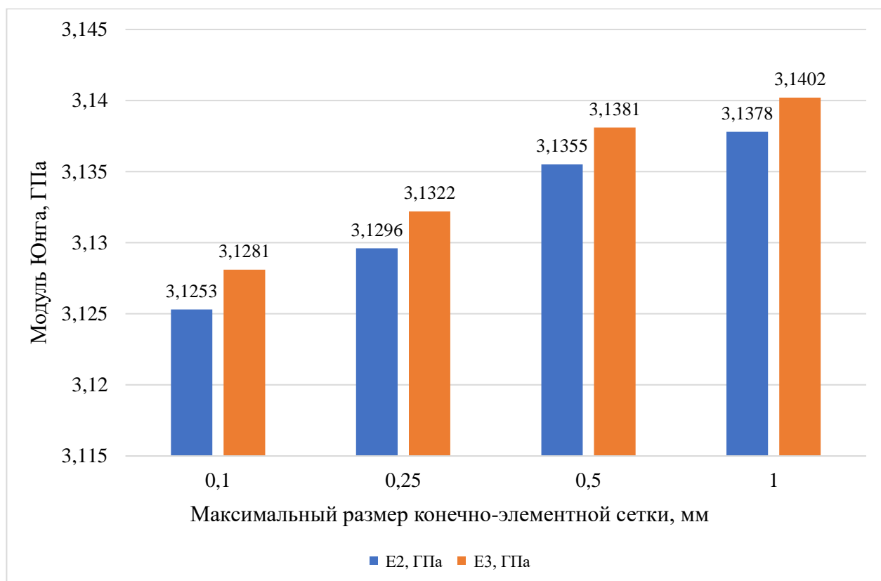
Рис.1.4.3. Изменение модуля Юнга E_2 , E_3 в зависимости от размера сетки
