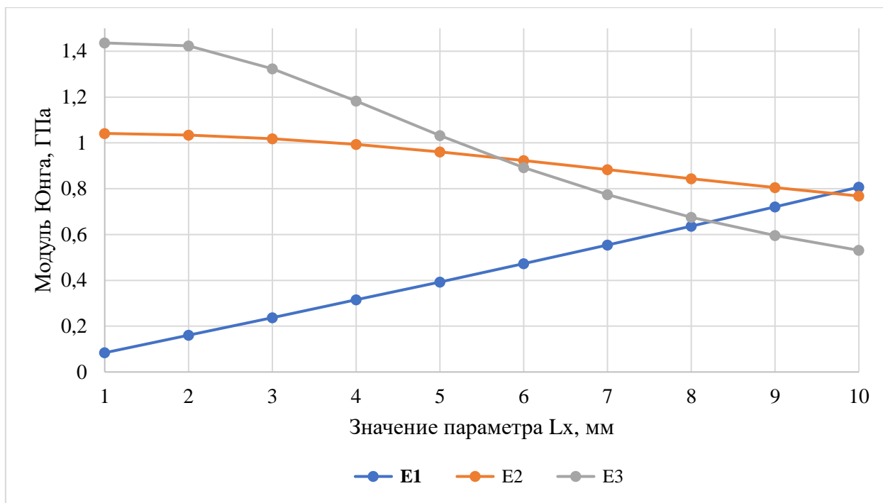
Рис.1.5.3.16. Зависимость значений модулей Юнга от параметра L_x для ячейки типа 5
