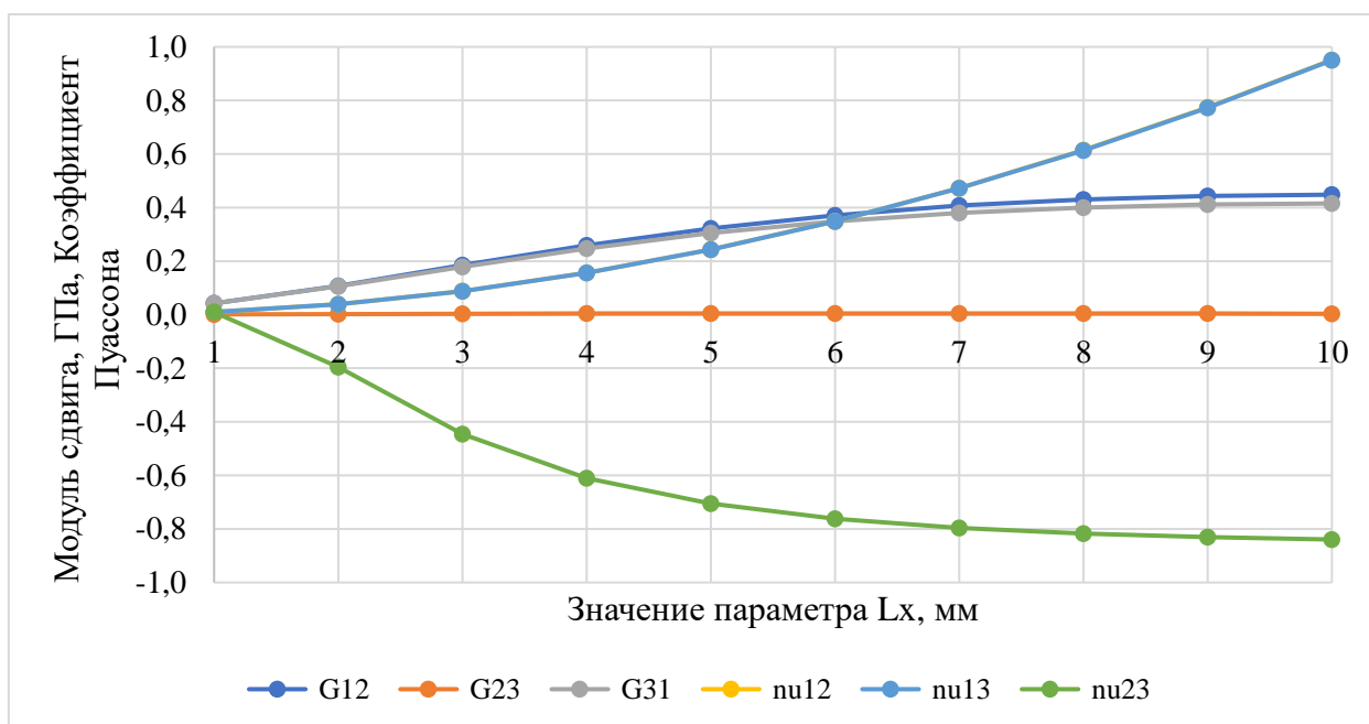
Рис.1.5.3.19. Зависимость значений модулей сдвига и коэффициентов Пуассона от параметра L_x для ячейки типа 6
