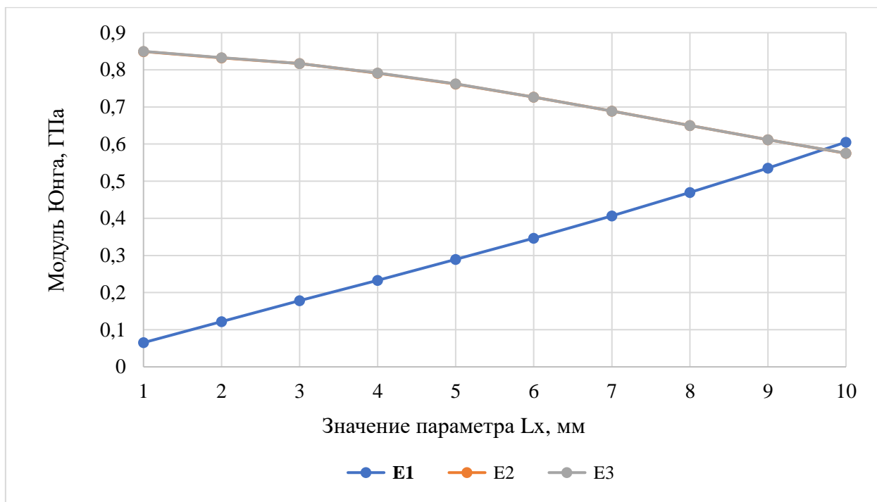
Рис.1.5.3.10. Зависимость значений модулей Юнга от параметра L_x для ячейки типа 2
