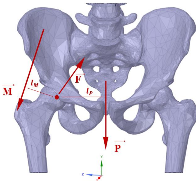
Рис.2.2.1.2. Схема нагружения модели таза. 1 сценарий нагружения
