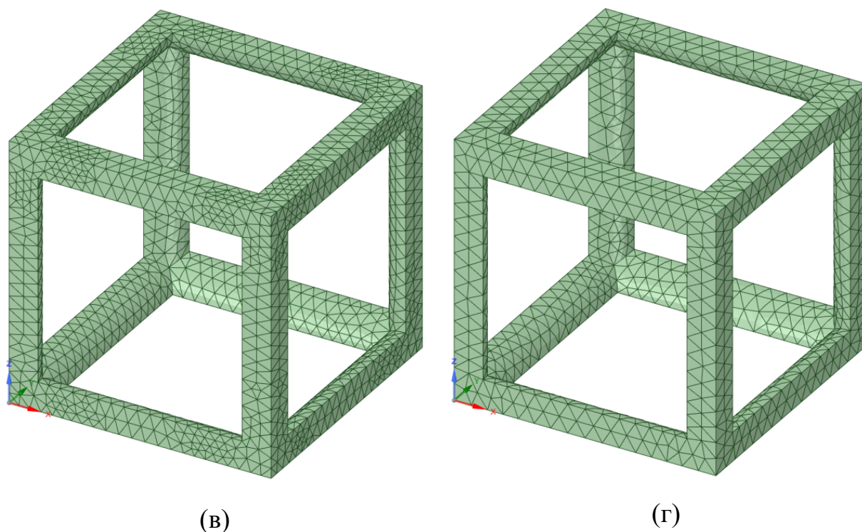
Рис.1.4.1. Внешний вид конечно-элементных моделей: (а) размер сетки 0,1 мм, (б) размер сетки 0,25 мм, (в) размер сетки 0,5 мм, (г) размер сетки 1 мм
