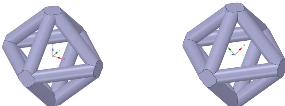
Рис.1.5.5.4. Внешний вид ячейки типа 4 до и после поворота локальных осей
