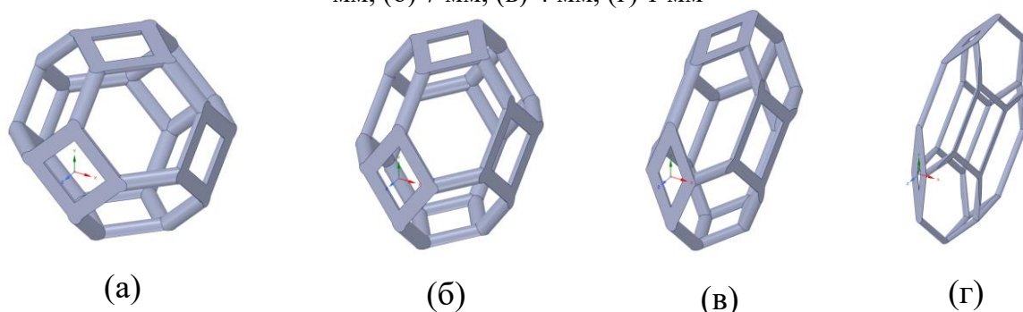
Рис.1.5.3.7. Внешний вид ячейки типа 7 при изменении геометрического размера L_x : (а) 10 мм, (б) 7 мм, (в) 4 мм, (г) 1 мм
