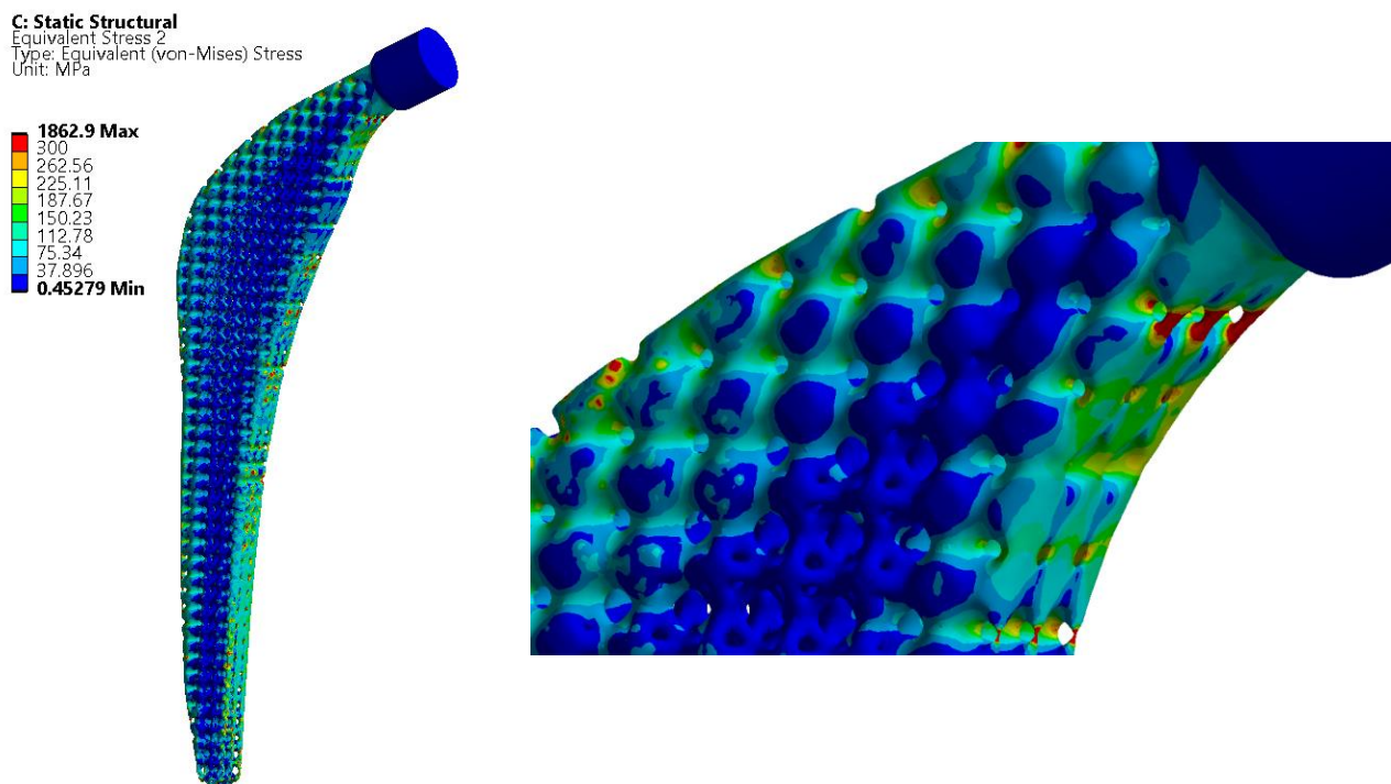
Рис.2.4.4. Эквивалентные напряжения (по Мизесу) компонента эндопротеза. 1 сценарий нагружения
