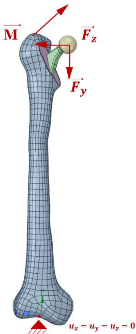
Рис.2.2.1.3. Нагрузки и ограничения, приходящиеся на рассматриваемую геометрию. 1 сценарий нагружения
