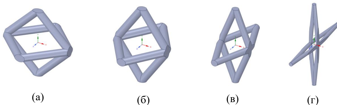
Рис.1.5.3.6. Внешний вид ячейки типа 6 при изменении геометрического размера L_x : (а) 10 мм, (б) 7 мм, (в) 4 мм, (г) 1 мм
