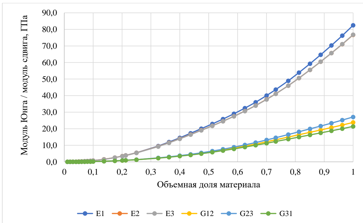
Рис.1.5.2.20. Зависимость значений модулей Юнга и модулей сдвига от объемной доли материала для ячейки типа 7
