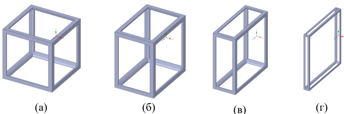
Рис.1.5.3.1. Внешний вид ячейки типа 1 при изменении геометрического размера L_x : (а) 10 мм, (б) 7 мм, (в) 4 мм, (г) 1 мм
