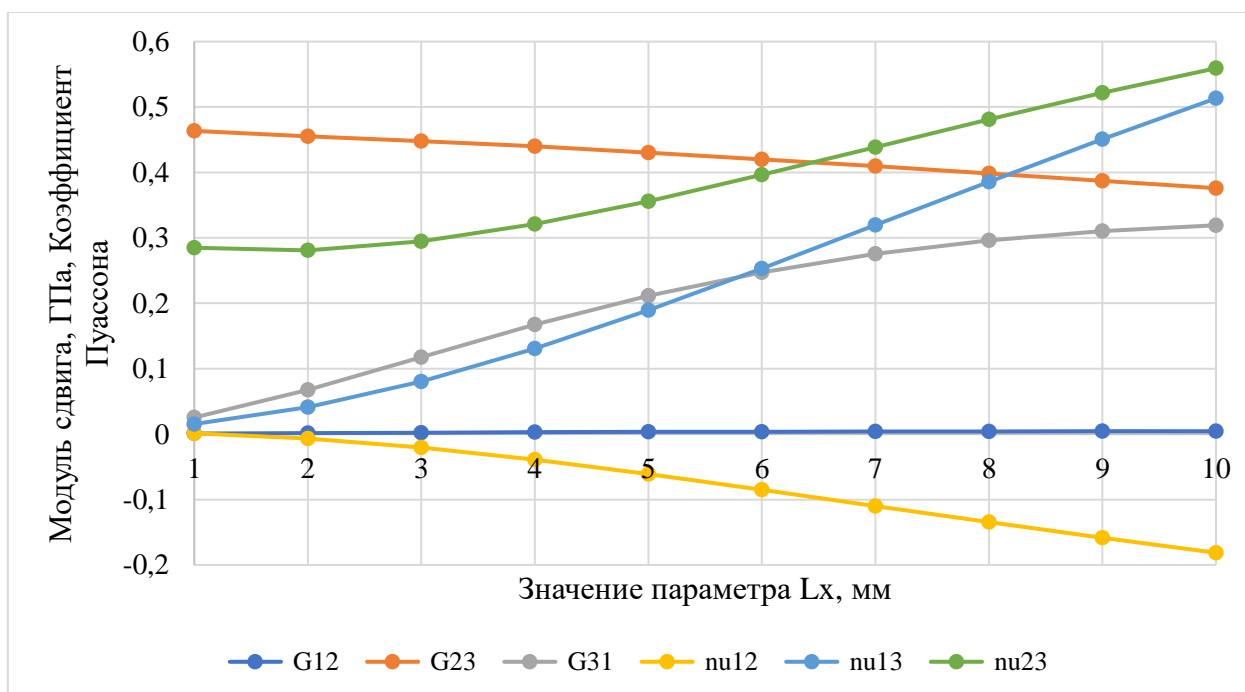
Рис.1.5.3.17. Зависимость значений модулей сдвига и коэффициентов Пуассона от параметра L_x для ячейки типа 5
