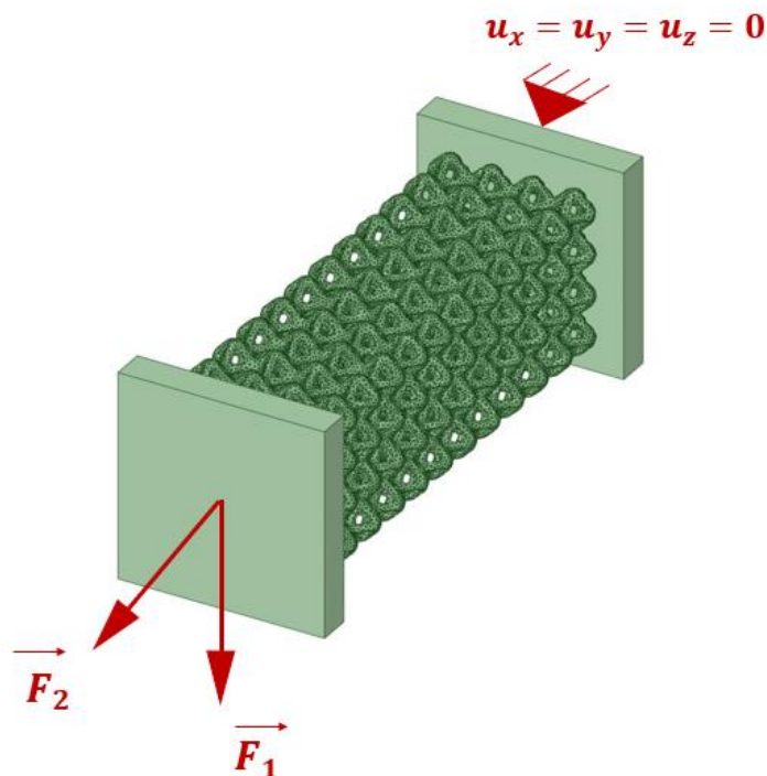
Рис.2.4.1. Схема нагрузок и ограничений, прикладываемых к модели для определения сеточной сходимости
