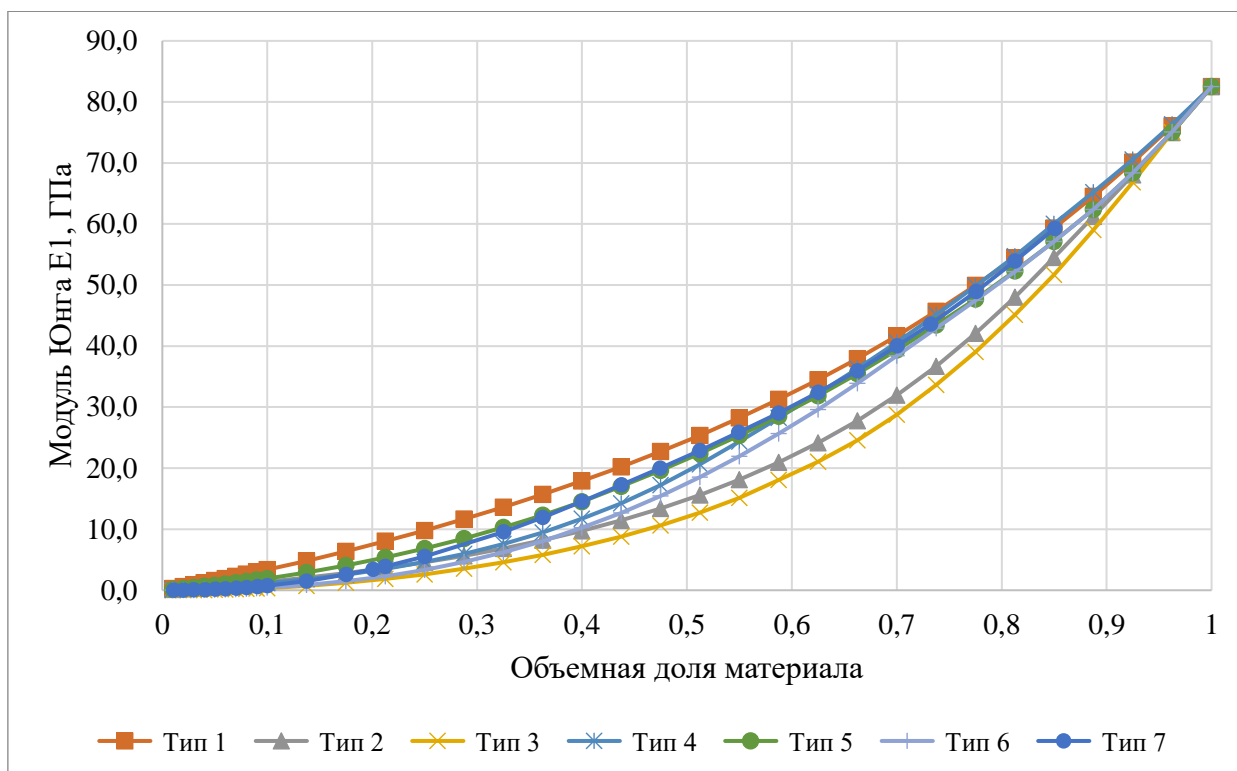
Рис. 1.5.2.22. Зависимость модуля Юнга E_1 от объемной доли материала для ячеек типов 1-7
