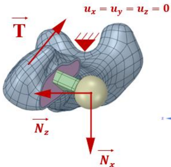
Рис.2.2.2.3. Нагрузки и ограничения, приходящиеся на рассматриваемую геометрию. 2 сценарий нагружения
