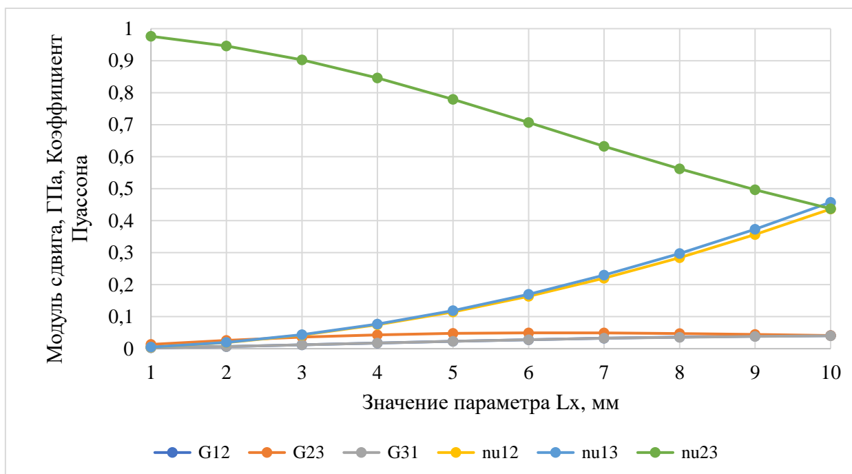
Рис.1.5.3.21. Зависимость значений модулей сдвига и коэффициентов Пуассона от параметра L_x для ячейки типа 7
