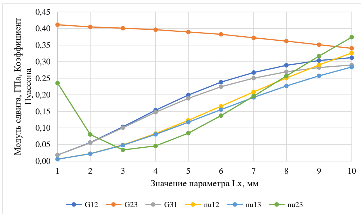
Рис.1.5.3.15. Зависимость значений модулей сдвига и коэффициентов Пуассона от параметра L_x для ячейки типа 4
