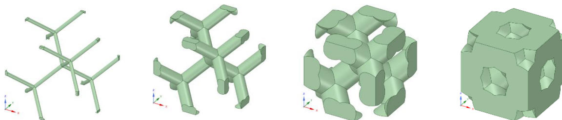
Рис. 1.5.2.2. Внешний вид ячейки типа 2 при различных значениях объемной доли материала: (а) 0,01; (б) 0,1; (в) 0,4; (г) 0,7
