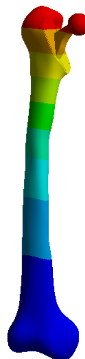
Рис.2.2.1.4. Распределение эквивалентных напряжений (по Мизесу) и модуля вектора перемещений для системы в случае 1 сценария нагружения
