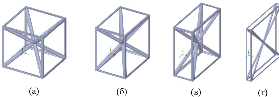
Рис.1.5.3.2. Внешний вид ячейки типа 2 при изменении геометрического размера L_x : (а) 10 мм, (б) 7 мм, (в) 4 мм, (г) 1 мм
