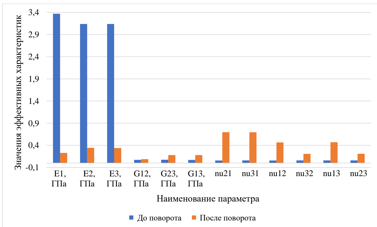
Рис.1.5.5.8. Значения эффективных характеристик до и после поворота локальных осей для элементарной ячейки типа 1
