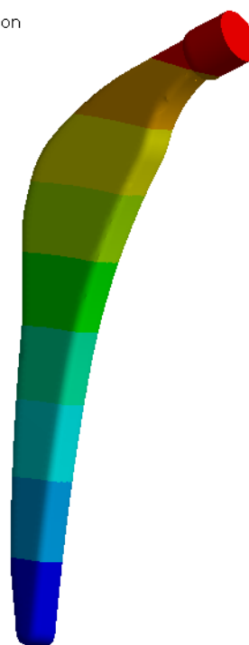
Рис.2.2.1.5. Распределение эквивалентных напряжений (по Мизесу) и модуля вектора перемещений для компонента эндопротеза в случае 1 сценария нагружения
