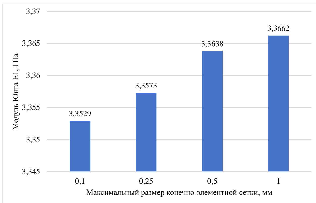
Рис.1.4.2. Изменение модуля Юнга E_1 в зависимости от размера сетки
