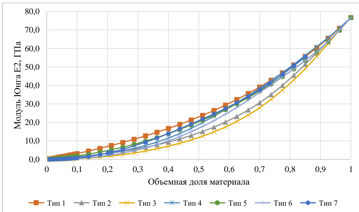
Рис.1.5.2.23. Зависимость модуля Юнга E_2 от объемной доли материала для ячеек типов 1-7
