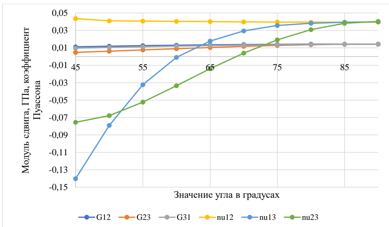
Рис.1.5.4.4. Зависимость модулей сдвига, коэффициента Пуассона от значений градусной меры угла между стержнями для ячейки типа 1
