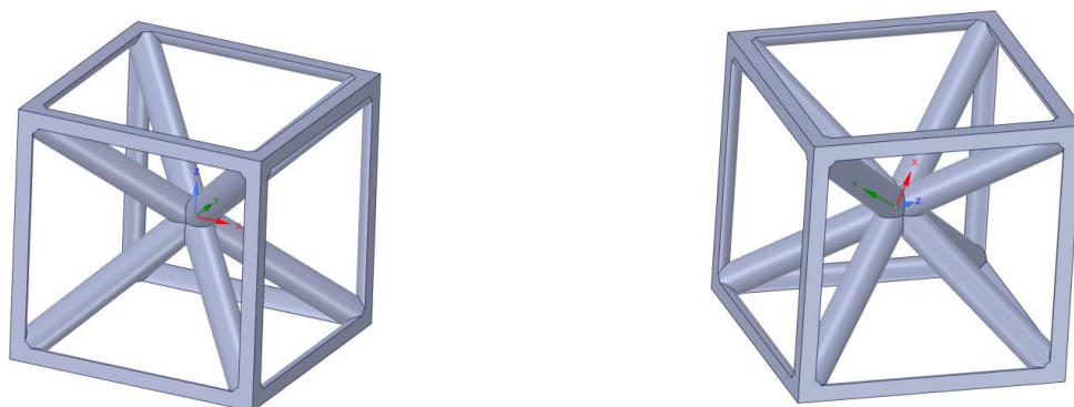
Рис.1.5.5.2. Внешний вид ячейки типа 2 до и после поворота локальных осей
