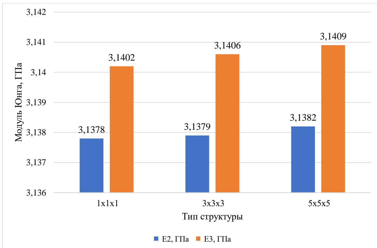
Рис. 1.4.6. Изменение значений модулей Юнга E_2 , E_3 в зависимости от размера периодической структуры
