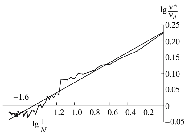
Рис. 2. Зависимость относительной откольной скорости от обратной толщины ударника (компьютерное моделирование).
