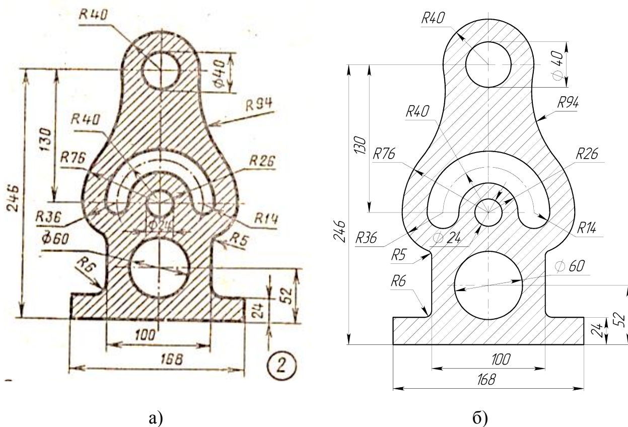
Рисунок 2. Стойка: а – задание; б – готовый эскиз детали
