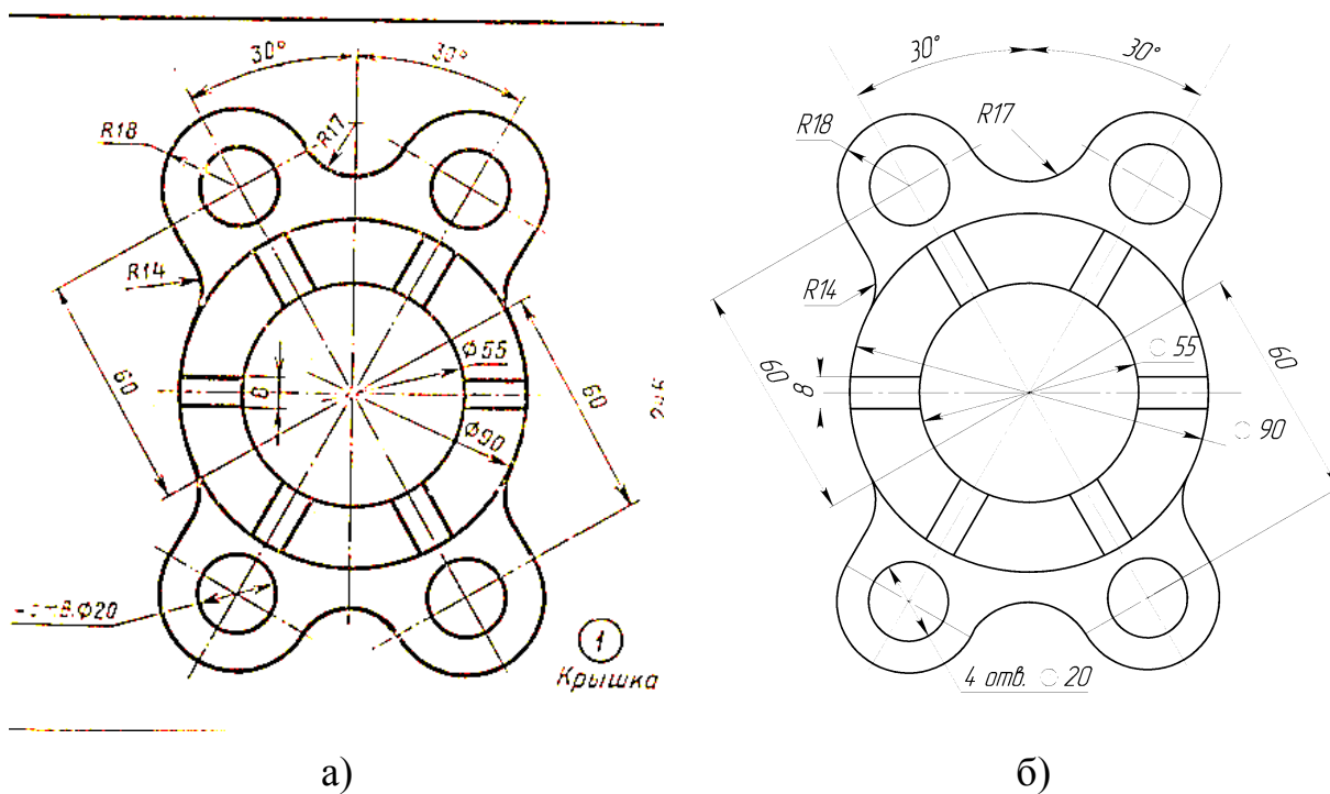
Рисунок 1. Подвеска: а – задание; б – готовый эскиз детали
