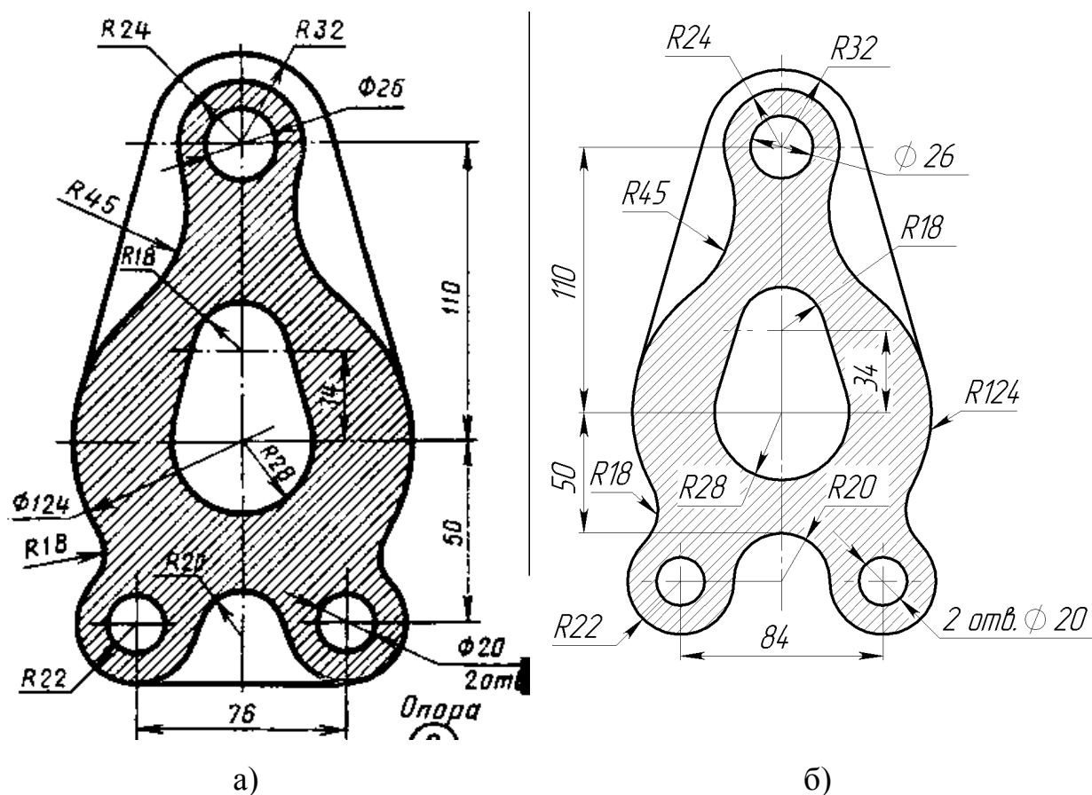
Рисунок 2. Корпус: а – задание; б – готовый эскиз детали
