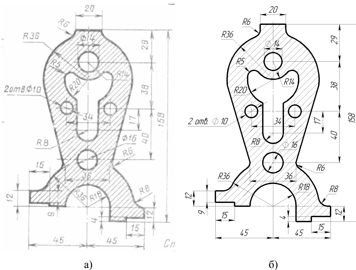
Рисунок 2. Стойка: а – задание; б – готовый эскиз детали
