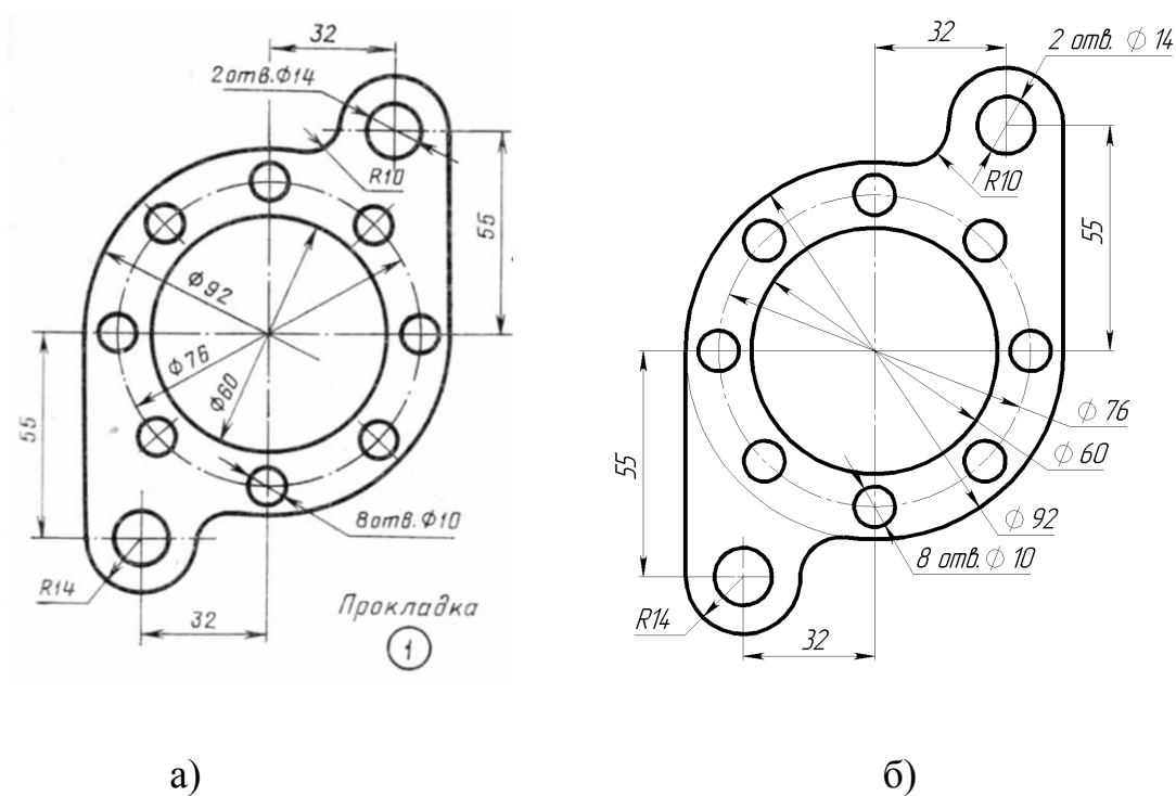
Рисунок 1. Прокладка: а – задание; б – готовый эскиз детали
