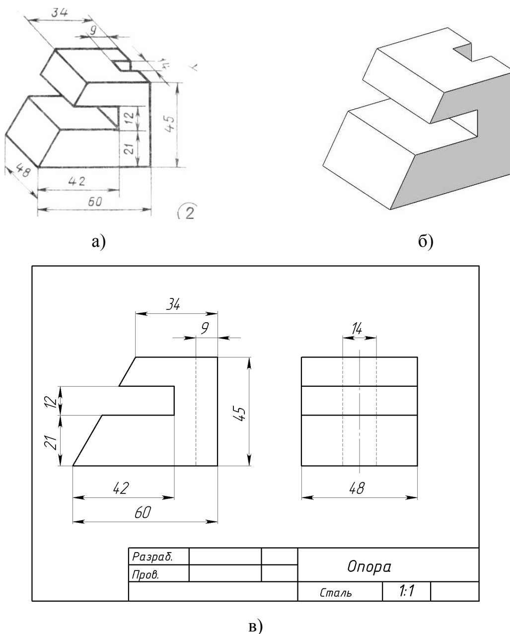
Рисунок 4. Опора: а – задание; б – готовая деталь; в – чертеж
