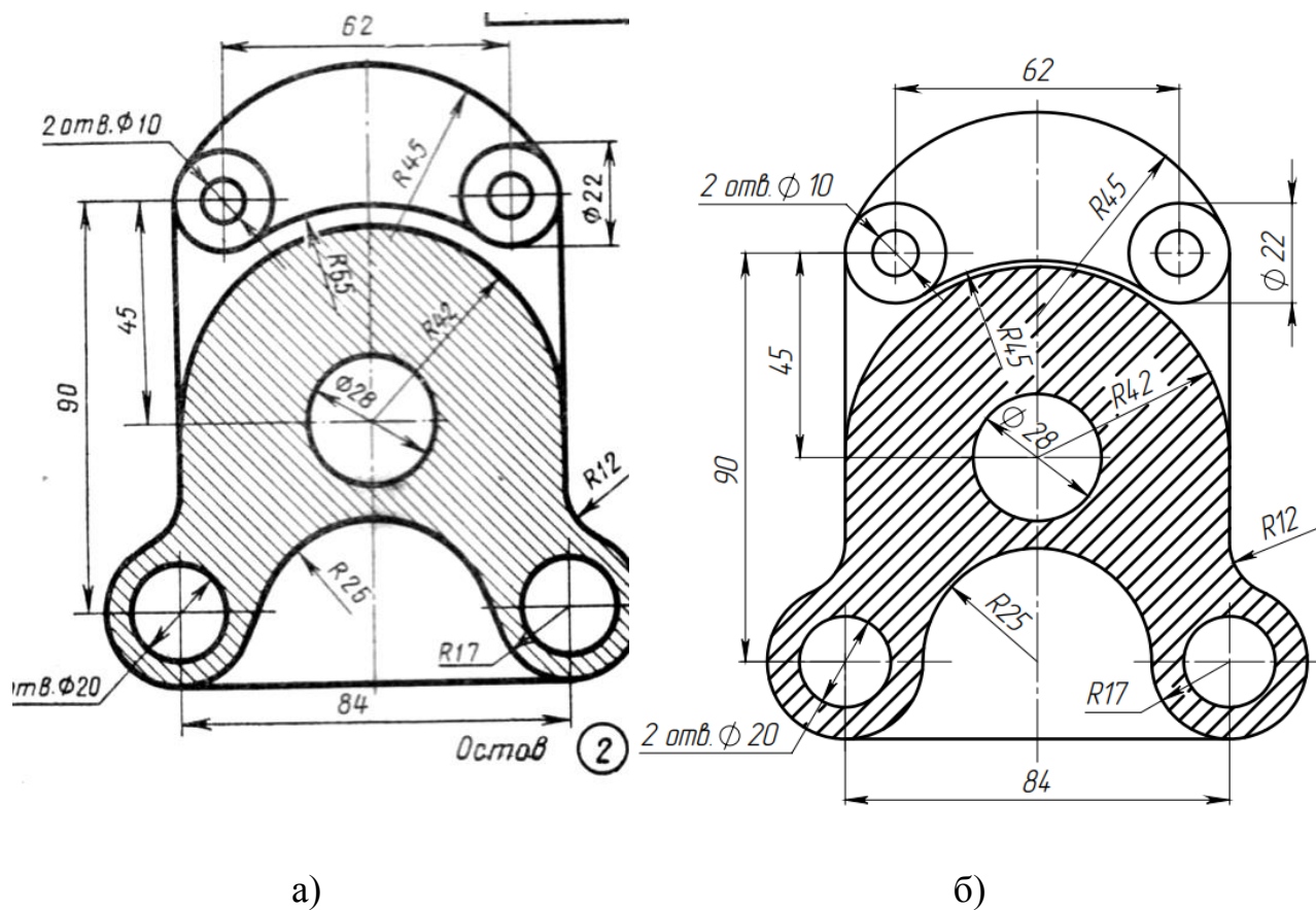
Рисунок 2. Остов: а – задание; б – готовый эскиз детали
