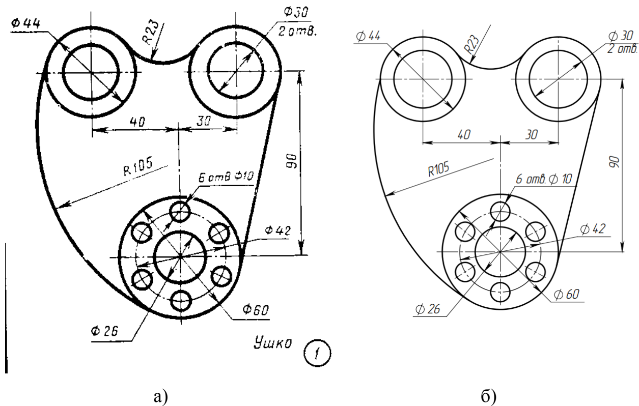
Рисунок 1. Ушко: а – задание; б – готовый эскиз детали
