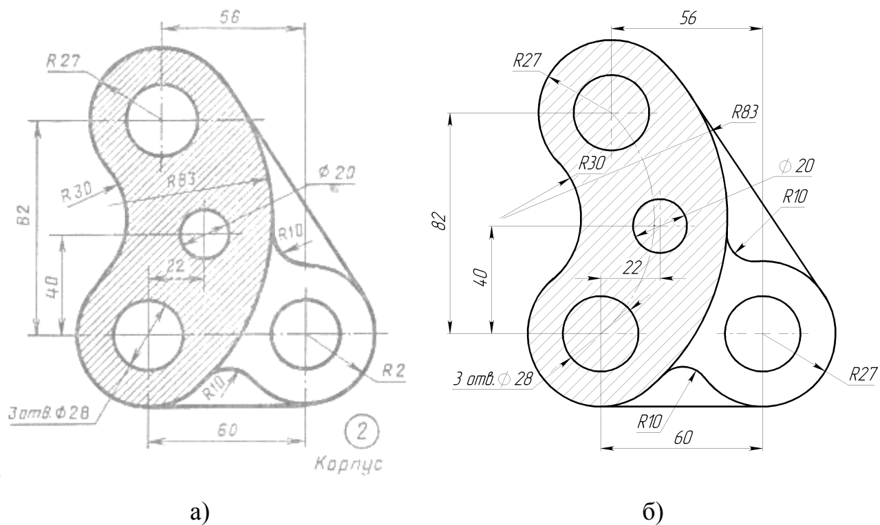
Рисунок 2. Корпус: а – задание; б – готовый эскиз детали
