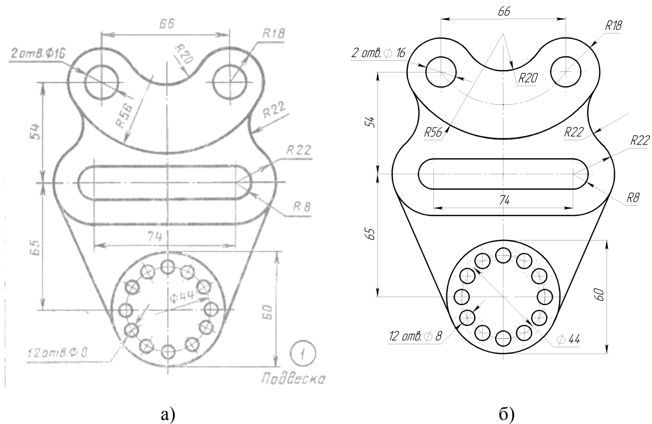
Рисунок 1. Подвеска: а – задание; б – готовый эскиз детали
